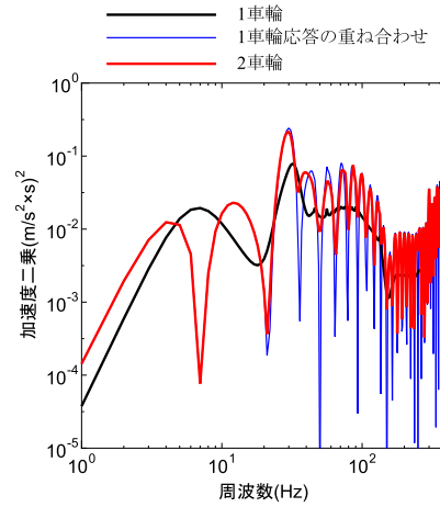
図 3 一車輪走行と二車輪走行の比較
