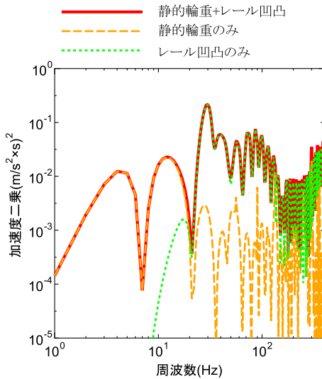
図 2 静的輪重およびレール凹凸の影響
