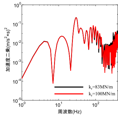
図 4 k_r の影響
