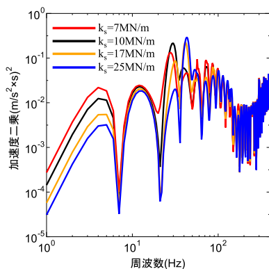
図 6 k_s の影響
