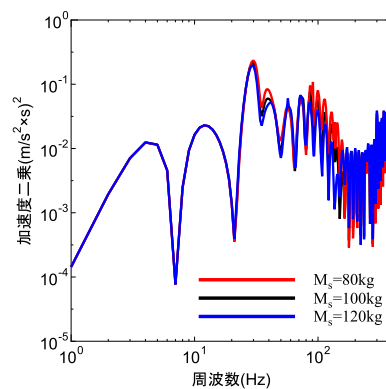
図 8 M_s の影響
