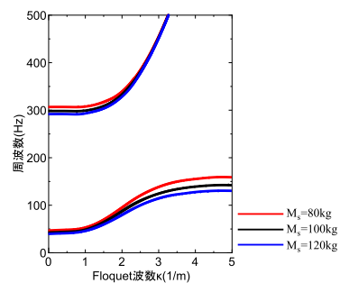
図 9 分散曲線が M_s に及ぼす影響
