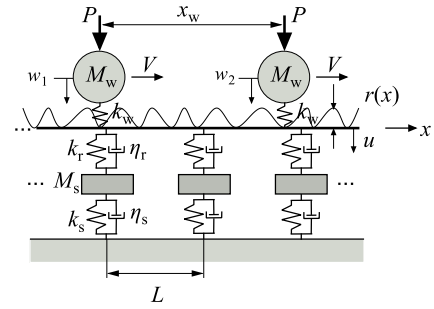
図 1 車輪・軌道連成系のモデル化
