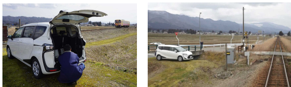
図7 実列車走行実験の状況(列車及び模擬停滞自動車)
