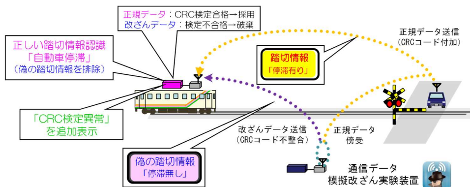
図5 模擬的な「なりすまし妨害」の対策
