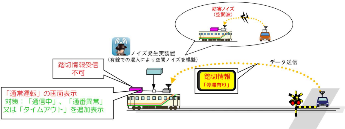
図 3 模擬的な「ノイズ妨害」の概要と対策
