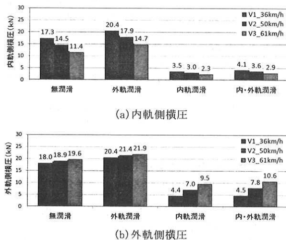
図 9 通過速度が異なる場合 (曲線半径 200m)
