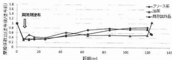
(b) 外軌側
