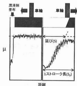
図2 延び性の評価法
