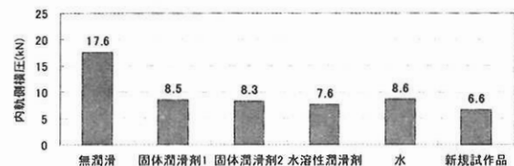
(a) 内軌側横圧
