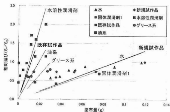
図3 各種潤滑剤の塗布量と相対延びの関係
