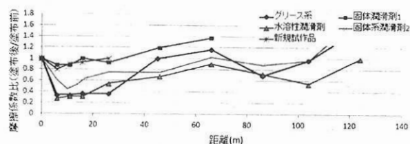
(a) 内軌側
