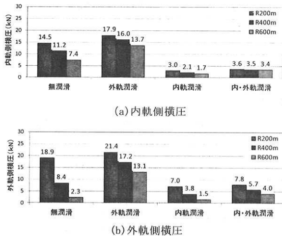
図 8 曲線半径が異なる場合 (均衡速度)
