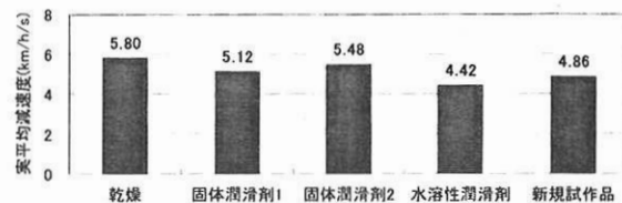
(a) 乾燥条件
