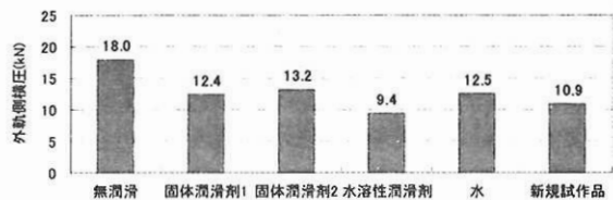
(b) 外軌側横圧
