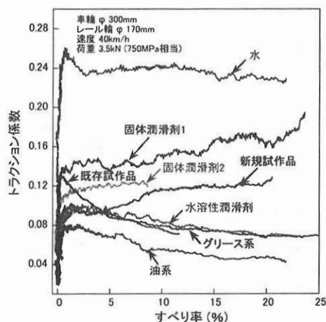
図1 各種潤滑剤のトラクション特性
