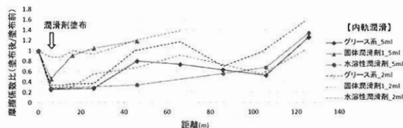
図5 潤滑剤の塗布量の違いによる伸び状況
