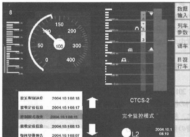
図-2 ATP車内ディスプレイの一例
