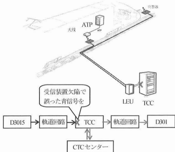
図3 CTCS-2システムのイメージ図
