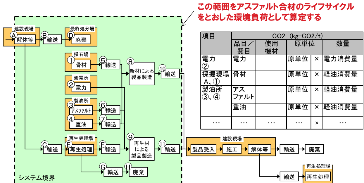
図-3 資材製造フロー及びシステム境界
