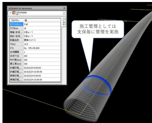
図6 支保単位の情報を表示
