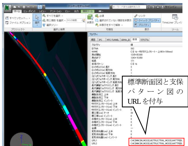
図4 トンネル本体の属性情報
