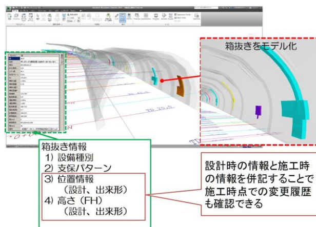
図7 電気設備情報を属性として表示
