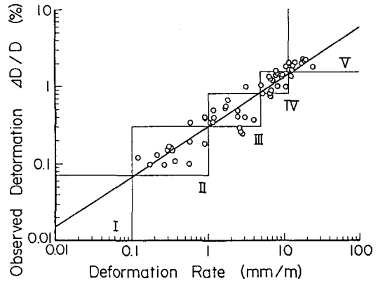
Fig. 5 初期変形率と観察された変形量との関係
