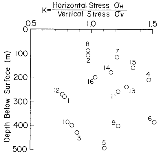
Fig. 2 水平方向応力と鉛直方向応力の比
