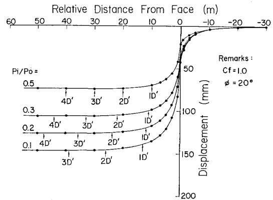
Fig. 3 数値解析から得たコンバージェンス曲線
