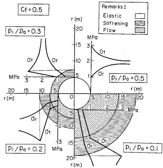
Fig.1 非弾性リングとグランドアーチ
