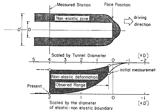
Fig. 4 コンバージェンス曲線の概念
