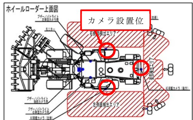
図-6 検知範囲図
