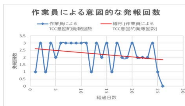
図-8 作業員による意図的な発報回数
