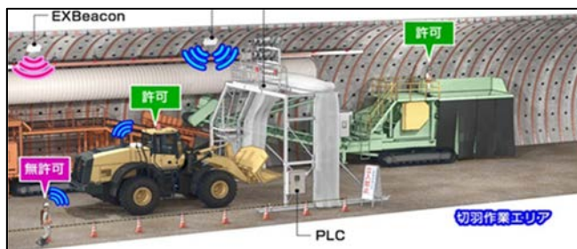
図-1 位置情報管理システム
