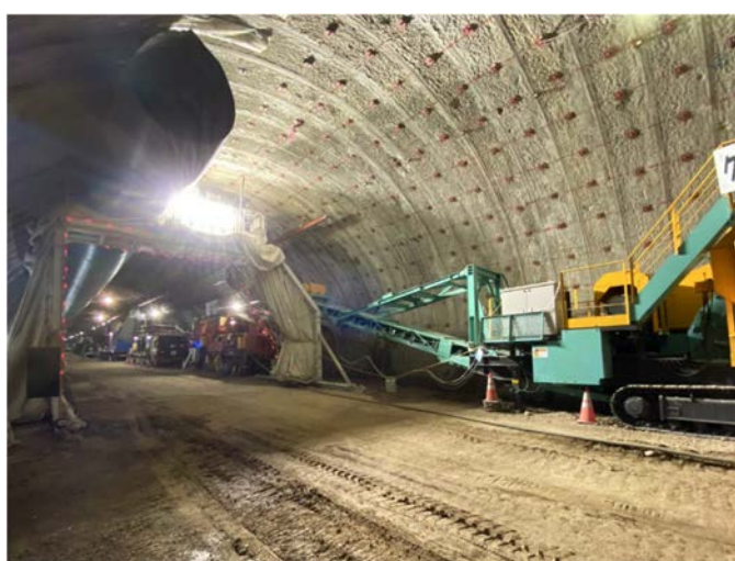
写真-3 照明架台と白色 LED 照明
