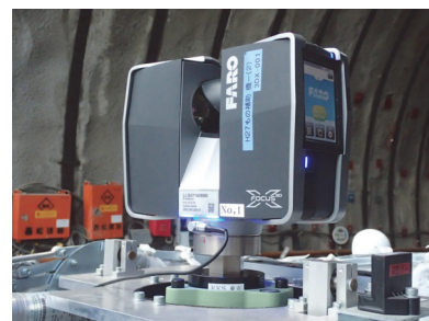
写真－2 3Dスキャナ外観
