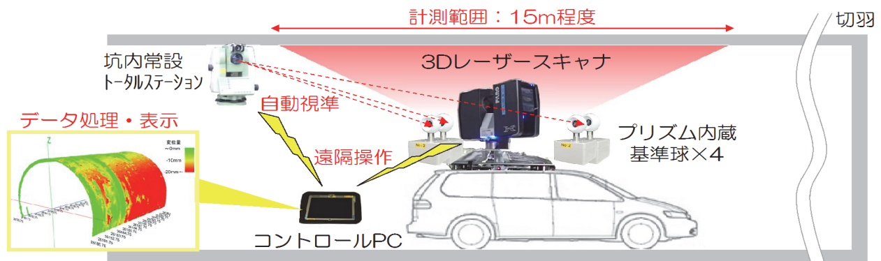
図-1 システム概要図
