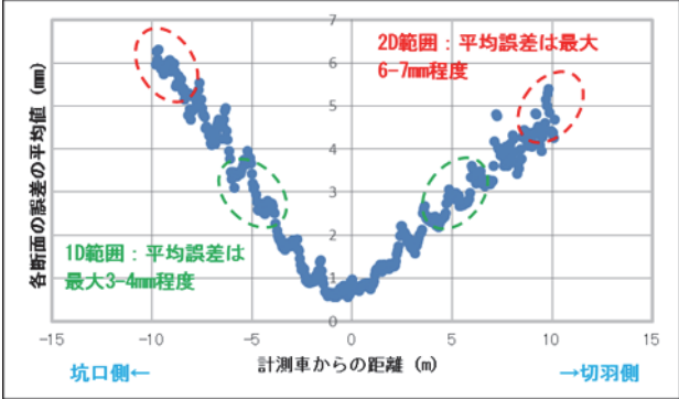
図－7 計測誤差の平均値と 計測車からの距離の関係
