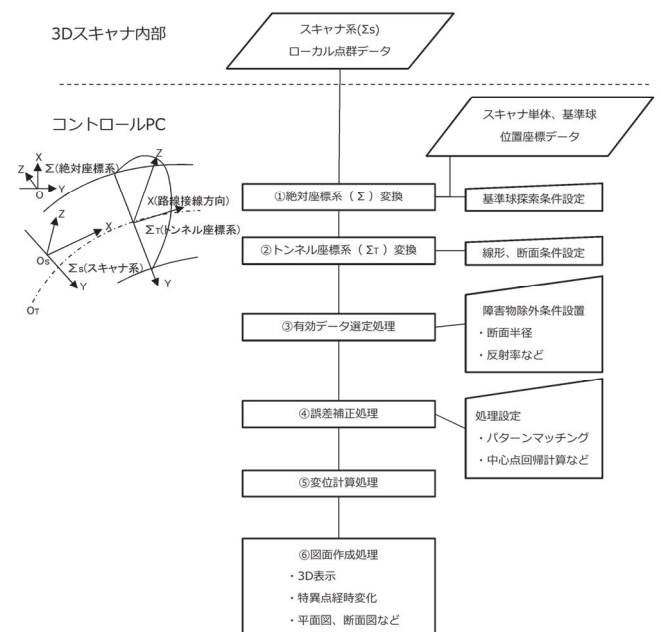
図－4 計測データ処理手順
