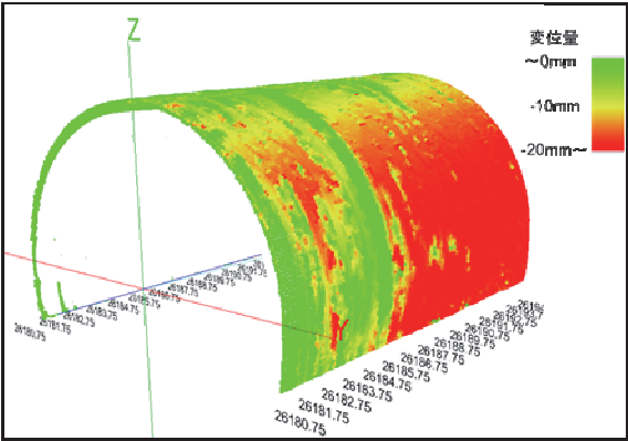
図－8 内空変位の計測結果(例)
