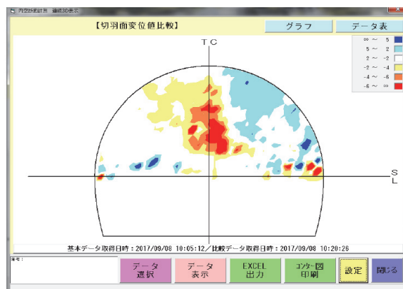
図－9 切羽面変位の計測結果(例)
