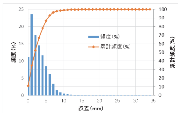
図-6 計測誤差の分布
