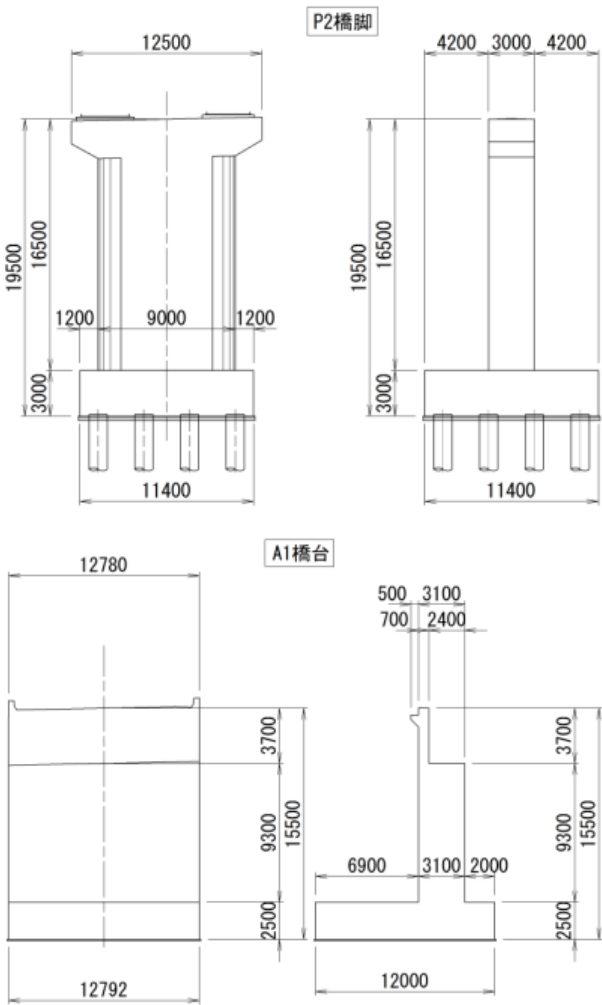
図－2 新小本大橋下部工構造図
