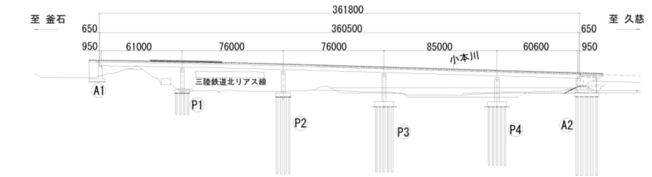
図－1 新小本大橋橋梁一般図
