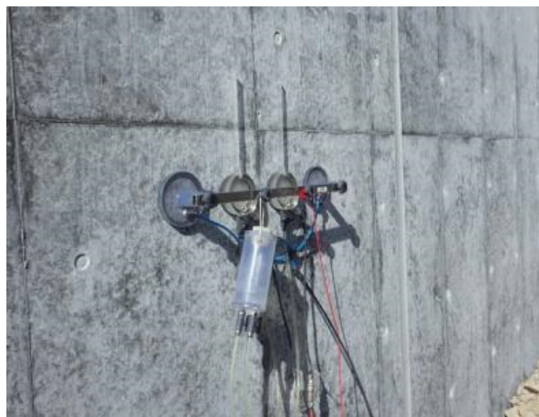
写真－7 SWAT 試験状況
