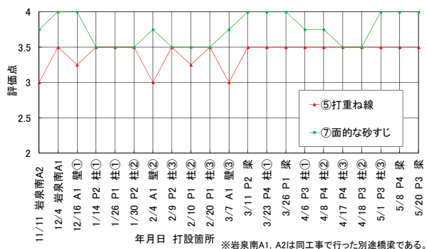
図－3 表層目視評価結果
