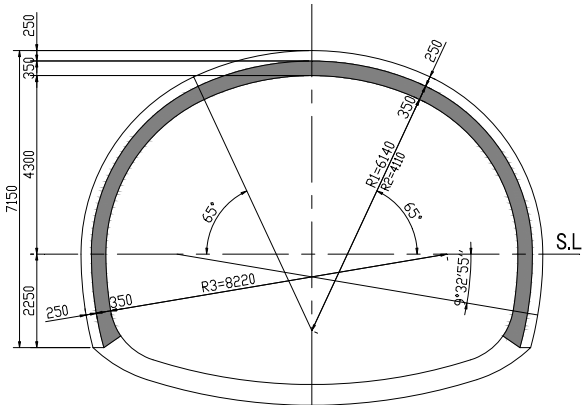
図-6 標準断面図(DⅢaパターン)の例
