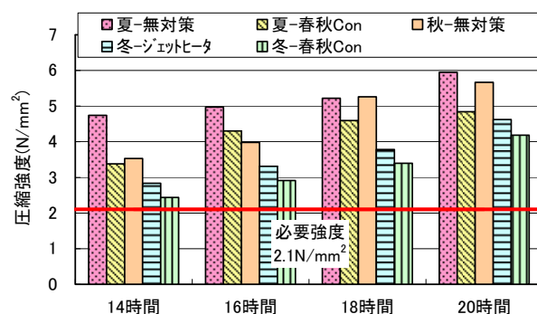
図-12 若材令強度試験結果
