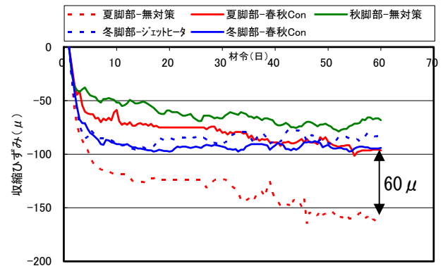
図-14 収縮ひずみ測定結果
