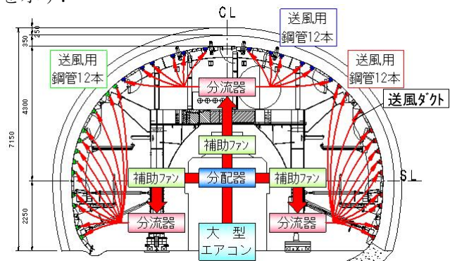
図-7 春秋コンクリート工法専用セントル概要図
