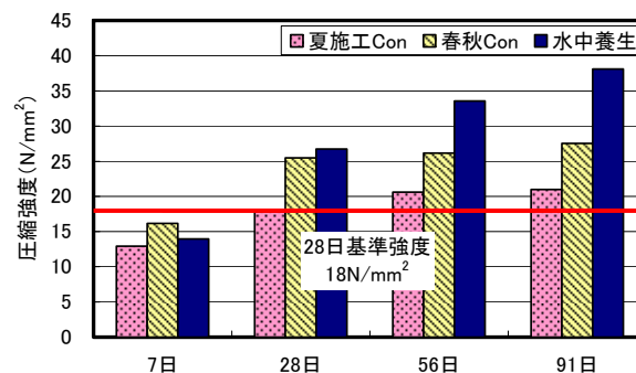
図-4 長期強度試験結果
