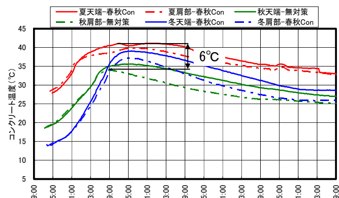
図-11 秋期施工のコンクリート中心温度比較
