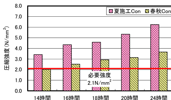
図-3 若材令強度試験結果
