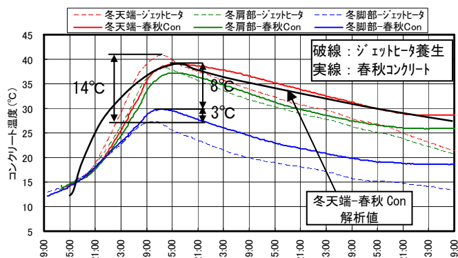
図-10 冬期施工のコンクリート中心温度比較
