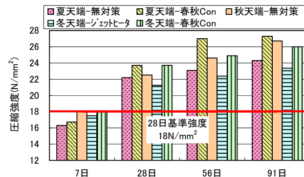
図-13 長期強度試験結果
