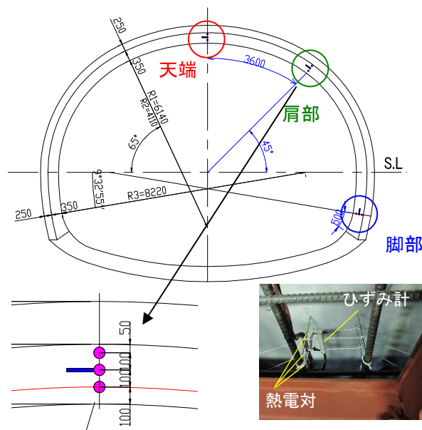
図-8 コンクリート温度および収縮ひずみ測定位置
