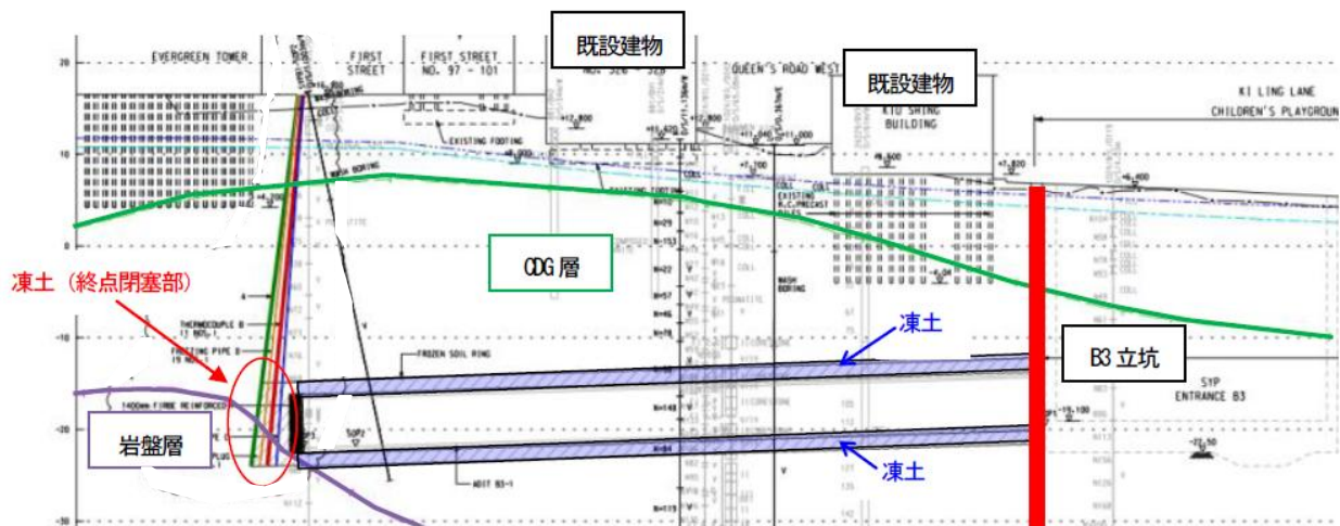
図－3 凍結横坑 B3 縦断面図
