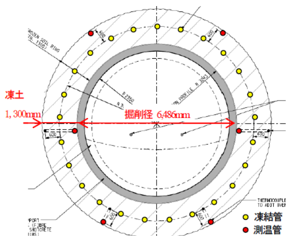
図-4 凍結横坑 B3 掘削断面図
