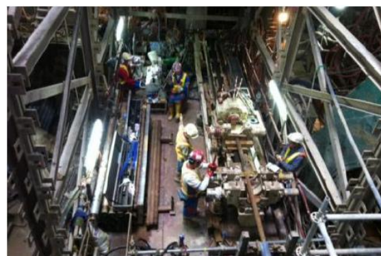
写真－1 水平コントロールボーリング施工状況
