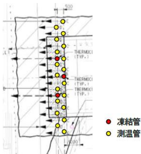
図-5 B3-1 閉塞部平面図
