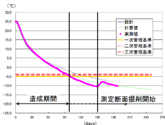
図－８ 地中温度測定グラフ
