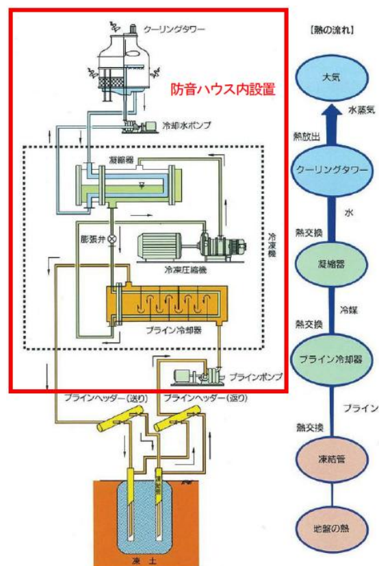
図－７ 凍結工フロー
