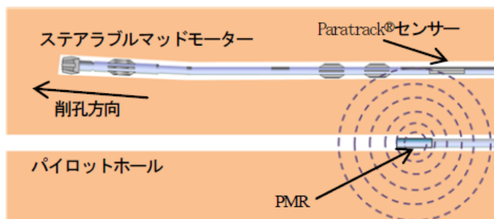
図－6 HDD システム概要図
