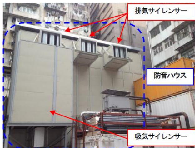
写真－２ 防音ハウス
