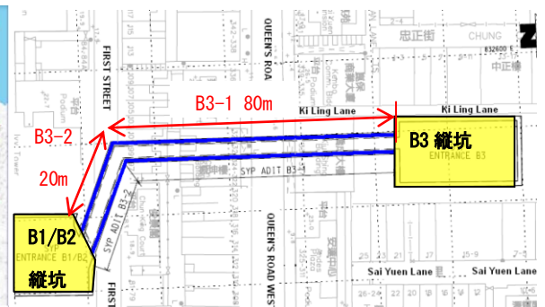
図－2 B3 横坑平面図
