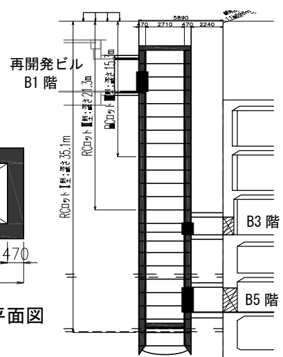
図-5 エレベーターシャフト断面図
