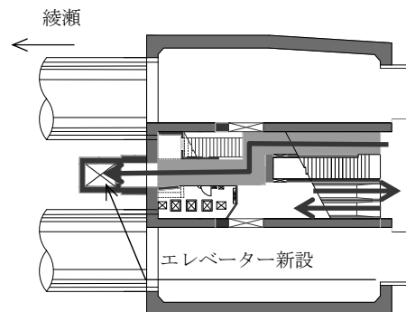
図-3 地下5階平面図
