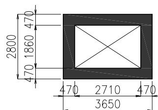
図-4 エレベーターシャフト平面図
