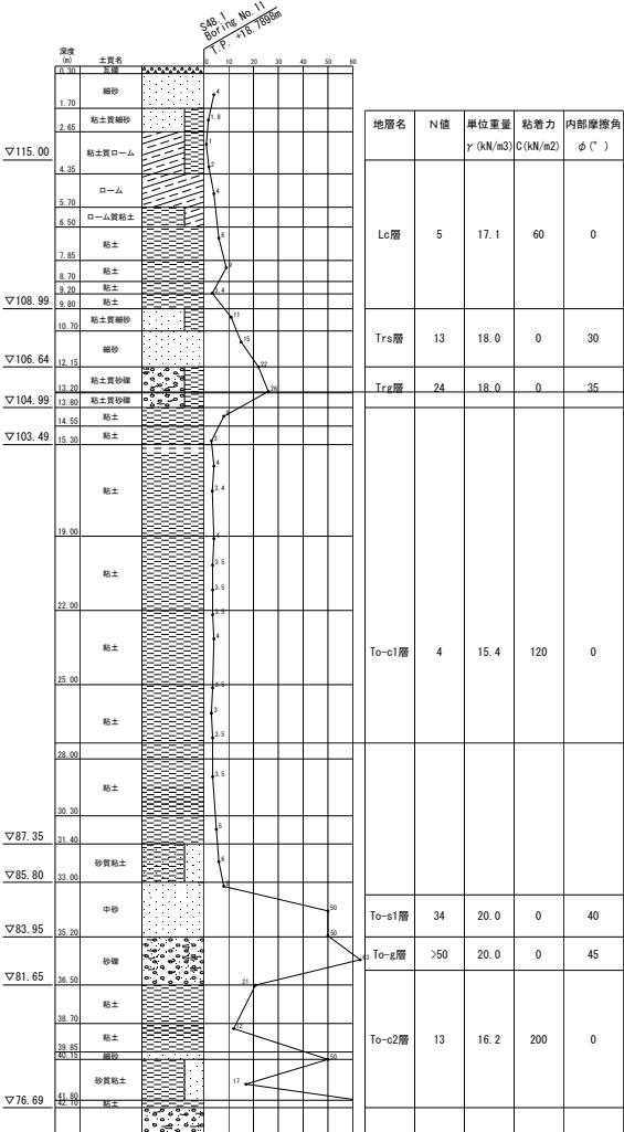
図-8 PC ウェル工 沈下関係図（必要圧入力）
