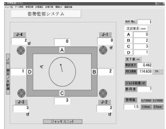
図-7 姿勢監視システム
