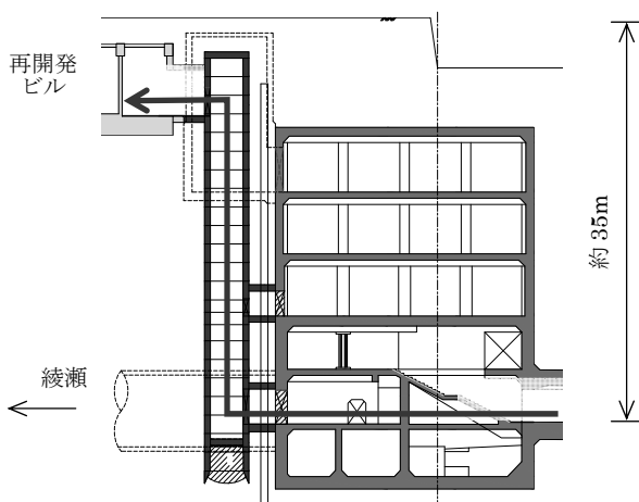
図-2 綾瀬方立坑断面図
