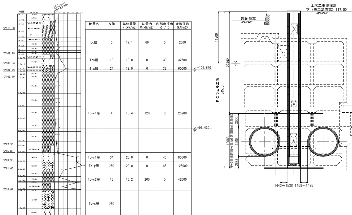
図-6 土質及びエレベーターシャフト位置図
