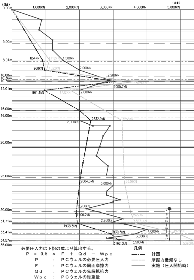
図-8 PC ウェル工 沈下関係図（必要圧入力）
