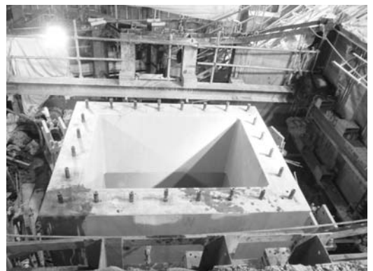
写真-3 施工完了
