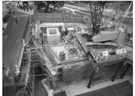
写真-2 施工状況（全景）
