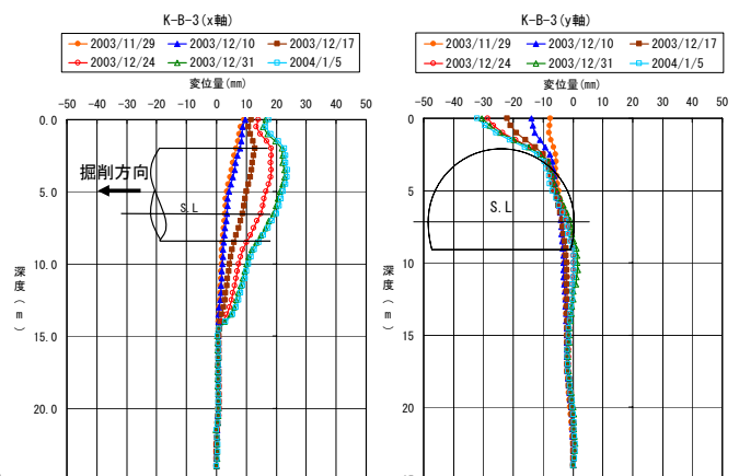
図-7 地中傾斜計計測結果
