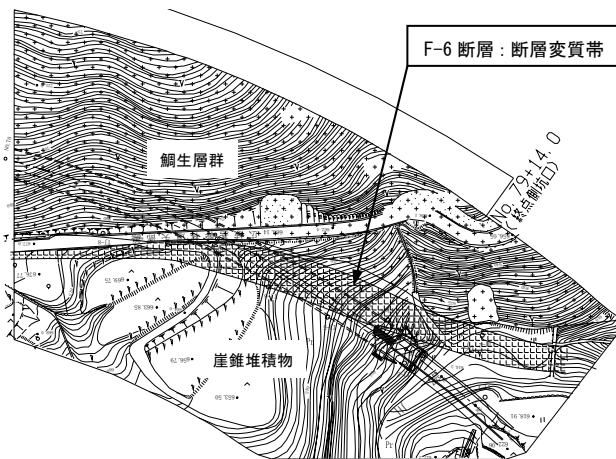
図-3 坑口部地質平面図
