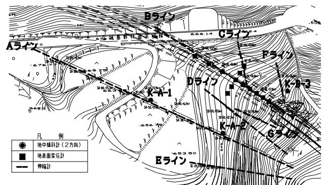
図-4 動態観測工配置図
