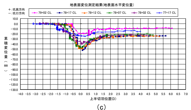
図-13 地表面変位測定結果
