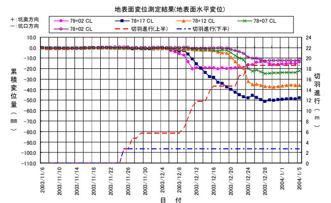
図-6 地表面変位測定結果
