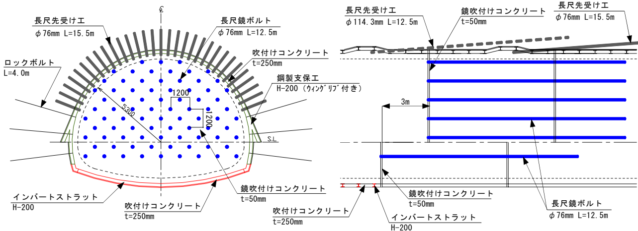
図-12 対策工の初期設定施工パターン
