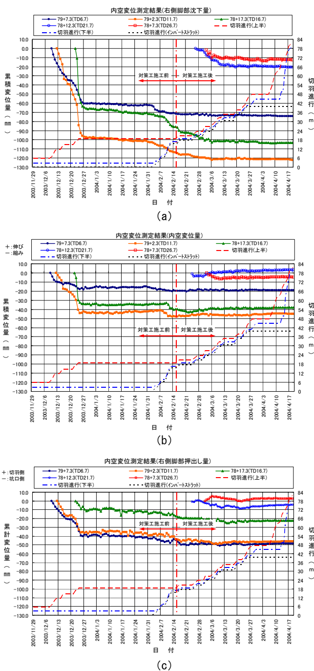
図-14 内空変位測定結果
