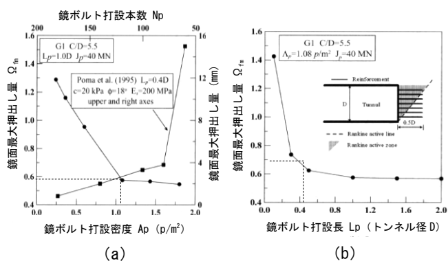
図-10 補強限界パラメーター 4)
