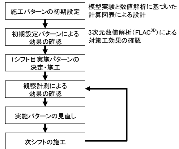
図-9 対策工の設計フロー
