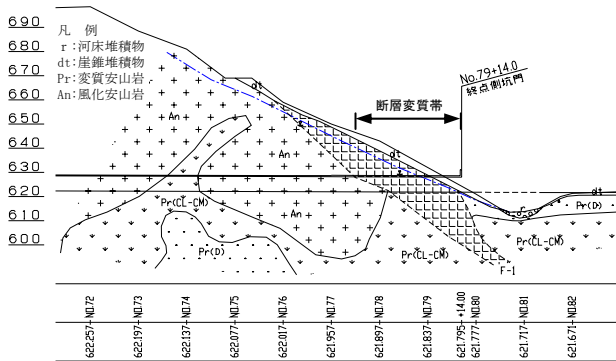
図-2 坑口部地質縦断面図
