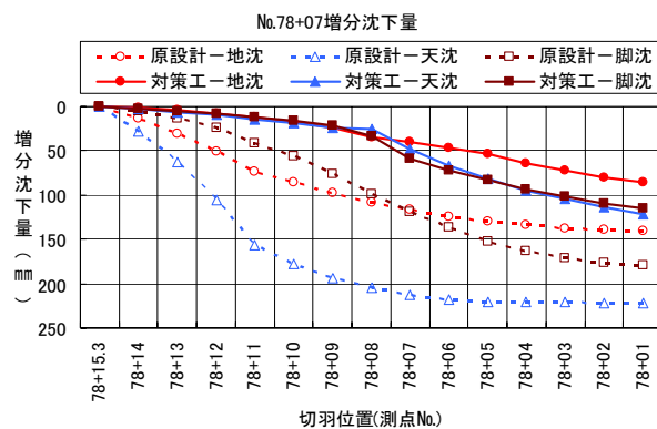
図-11 三次元数値解析による増分沈下量
