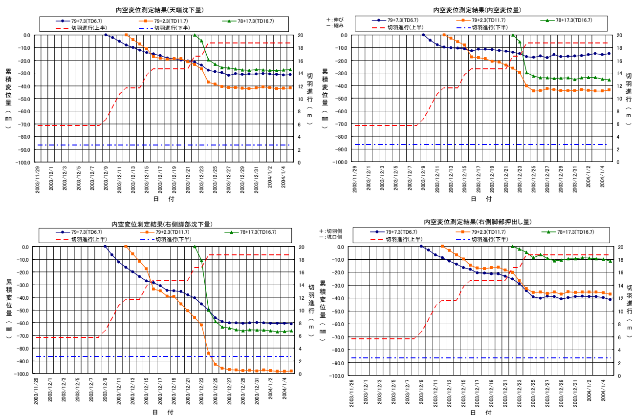
図-8 内空変位測定結果
