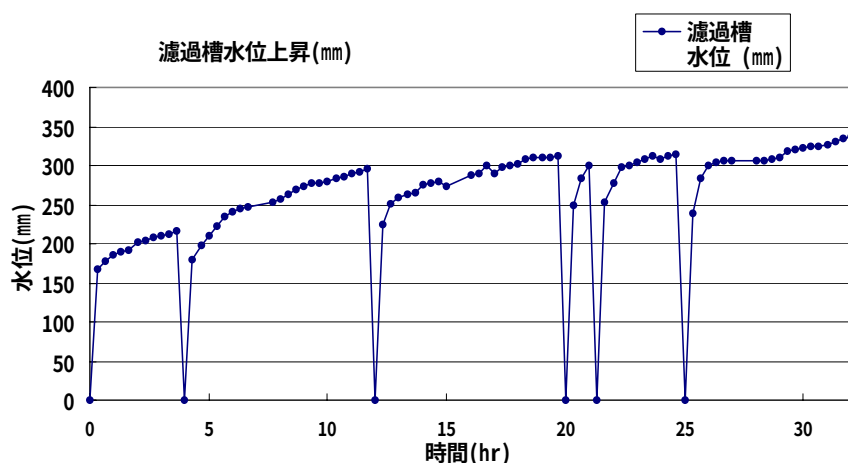
図-4 濾過槽水位の推移
