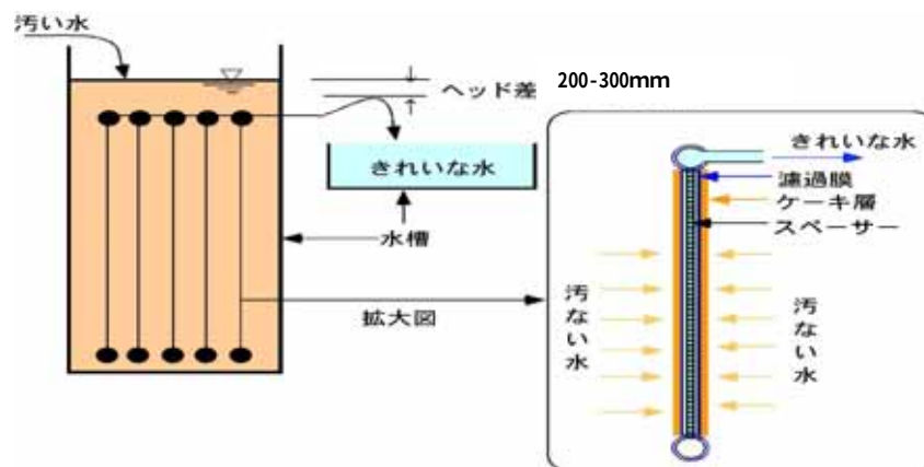
図-2 膜濾過の処理原理
