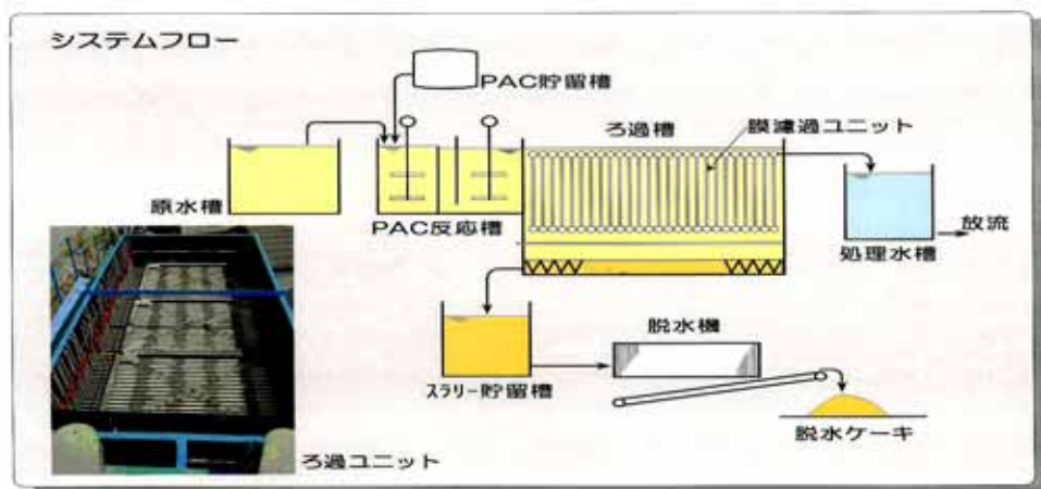
図-1 システムフロー
