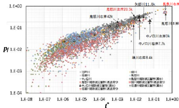
図-8 堤防脆弱性指標 t^* と破壊危険確率 P_f の関係
