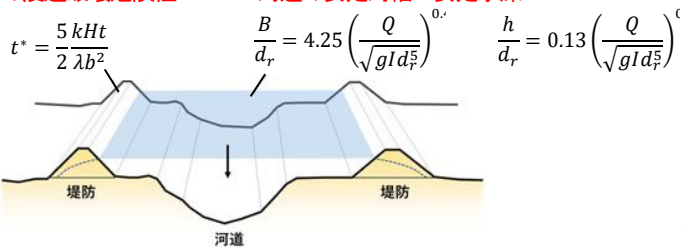
図-10 治水と環境の調和した河道計画，設計の考え方
