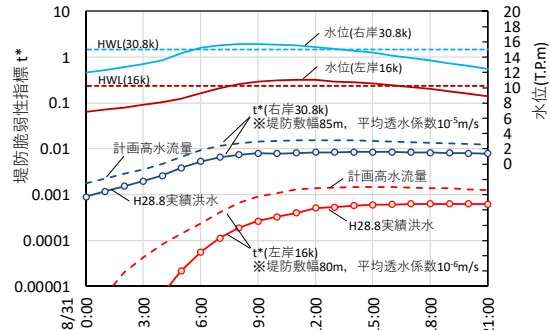
図-9 十勝川の洪水水位の時間変化に対する t^*
