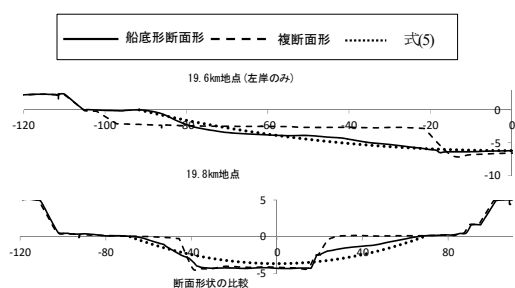
図-5 船底形河道断面形と式(5)の比較
