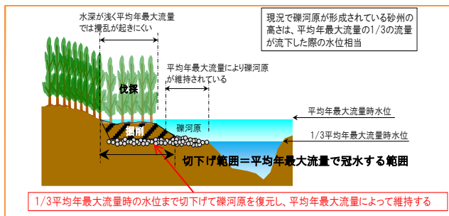
図-14 切下げ範囲・高さのイメージ図
