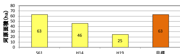
図-2 目標とする昭和60年代の礫河床面積
