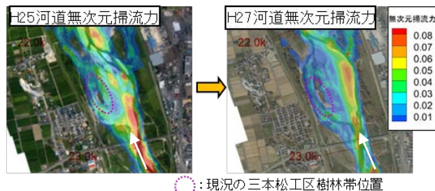
図-13 河道の違いによる無次元掃流力分布の変化
