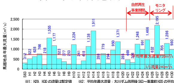
図-4 事業期間前後の馬越地点年最大流量
