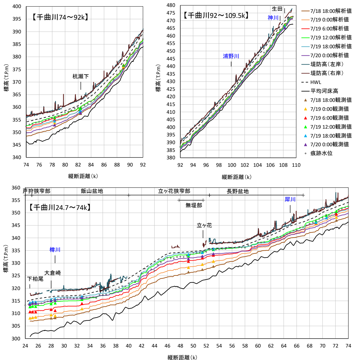
図-3 千曲川の水面形時間変化の観測値と解析値の比較
