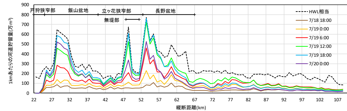
(a) 1km毎の河道貯留量縦断分布の時間変化
