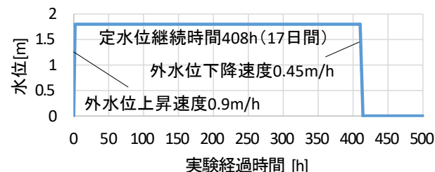
図-2 実験の外力条件
