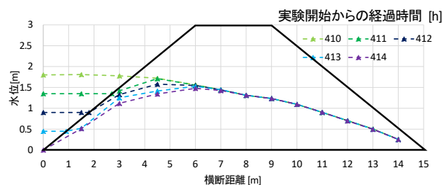
図-3 外水位降下時の堤体内浸潤線の観測値
