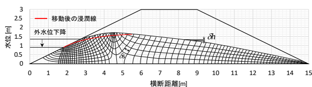
(a) 水位下降開始から2時間後の結果
