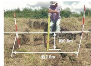
(b) 堤防裏法崩れ
