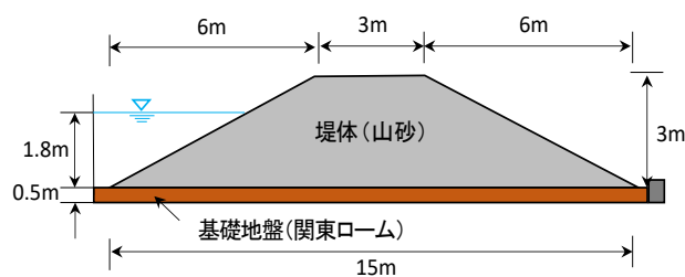
図-1 土木研究所大規模実験模型の断面形状
