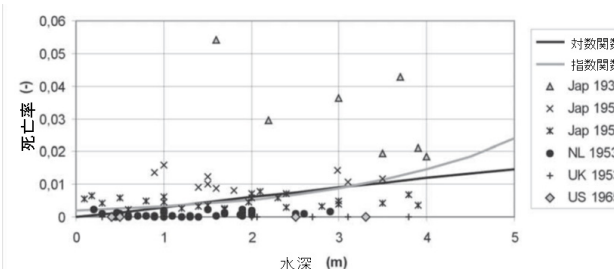
図-9 水深が支配的な【領域3】での死亡率 15)
