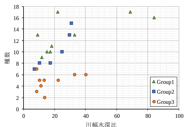
図-5 川幅水深比と種数の関係
