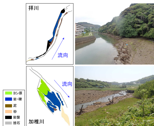
図-6 川幅の変化とハビタットの多様性
