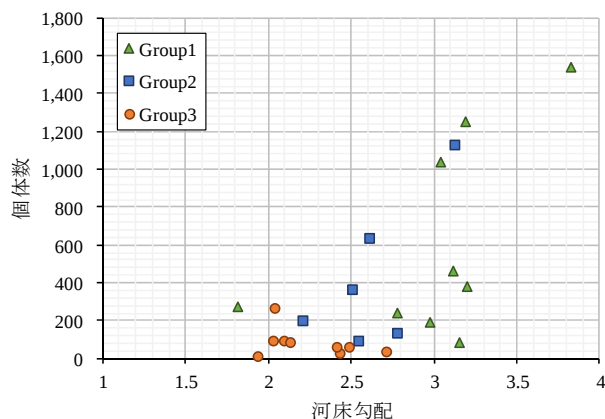
図-4 河床勾配と個体数の関係
