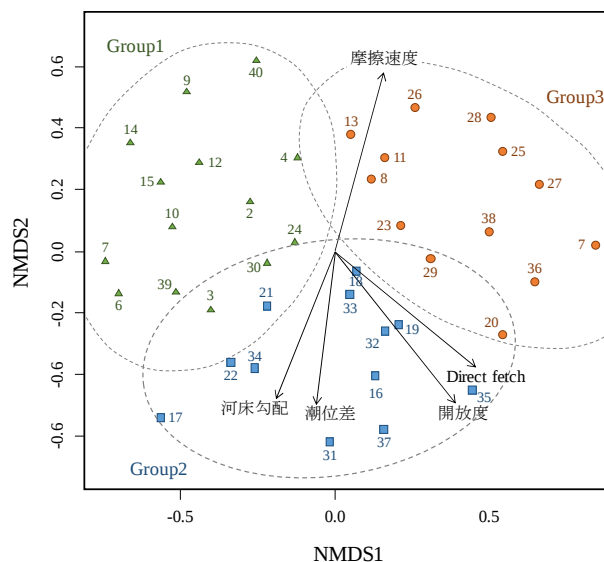
図-2 NMDSによる対象河川の貝類相の解析と物理要因
