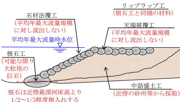
図-2 「巨石付き盛土砂州を用いた河岸防護工」の構造
