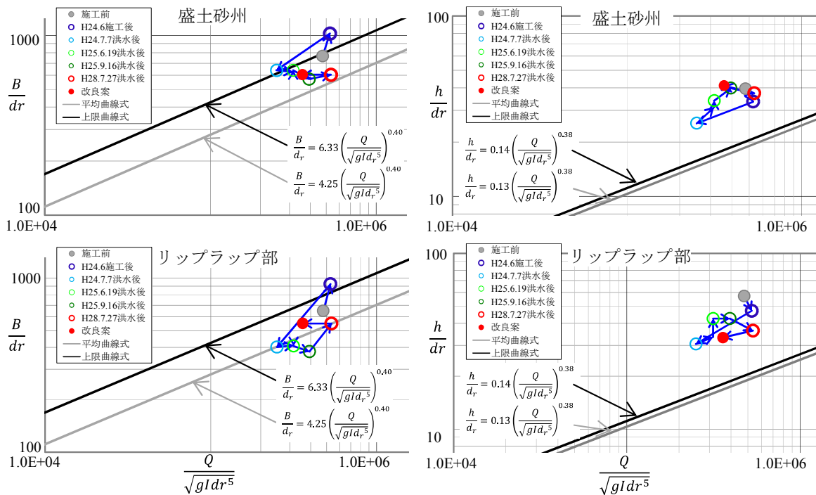
図-14 平均年最大流量（瓶岩地点700m³/s程度）流下時の無次元流量と無次元川幅、無次元水深の関係
