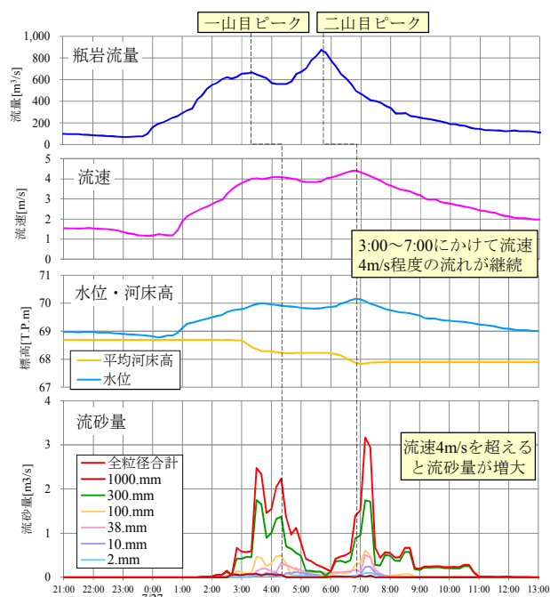
図-12 流況および河床変動の解析結果
