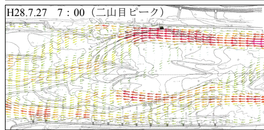
図-11 流速ベクトル図（H28.7.27洪水）
