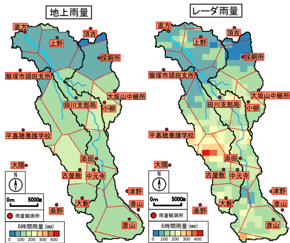
図-4 地上雨量とレーダ雨量の6時間雨量の空間分布
