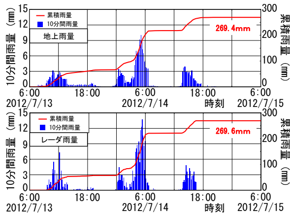
図-3 流域平均ハイエトグラフ
