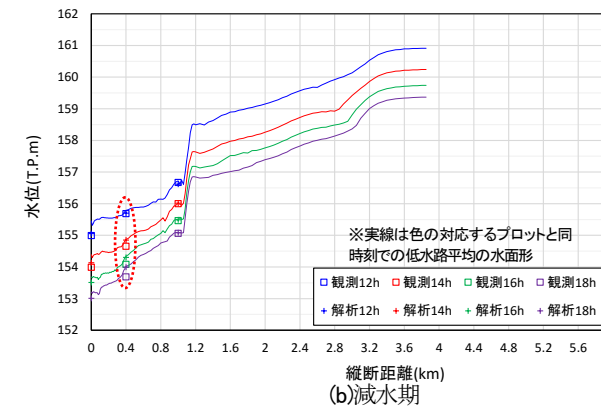
図-10 西城川の観測水面形と解析水面形の比較 (平成26年8月洪水)
