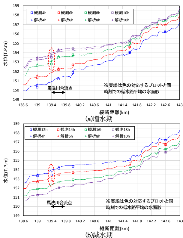
図-5 江の川の観測水面形と解析水面形の比較 (平成25年9月洪水)
