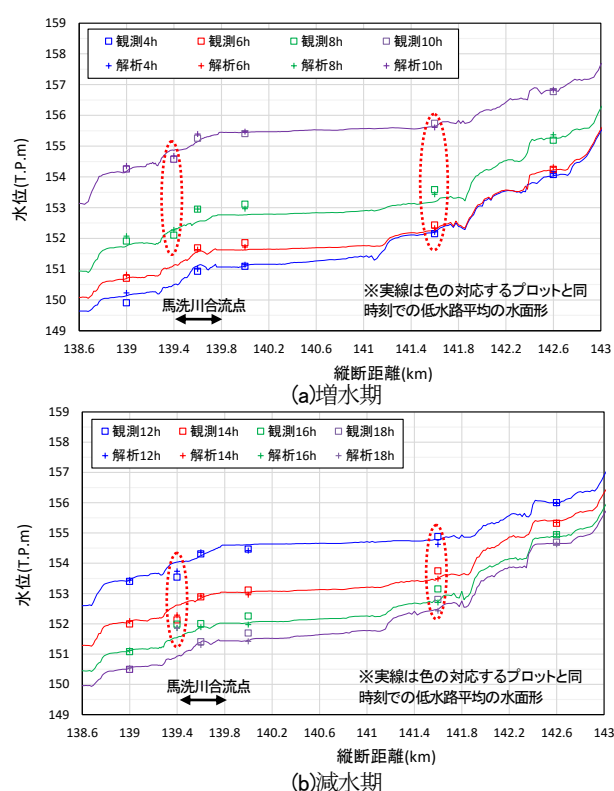
図-6 江の川の観測水面形と解析水面形の比較 (平成26年8月洪水)
