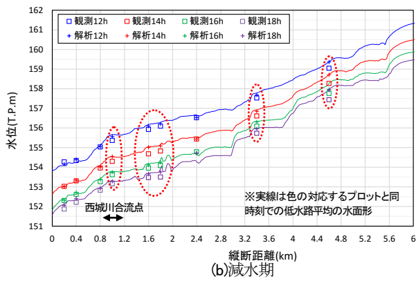
図-8 馬洗川の観測水面形と解析水面形の比較 (平成26年8月洪水)
