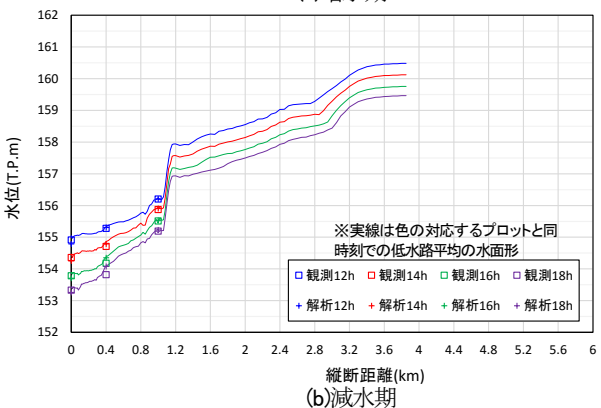
図-9 西城川の観測水面形と解析水面形の比較 (平成25年9月洪水)
