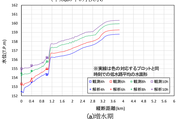
図-7 馬洗川の観測水面形と解析水面形の比較 (平成25年9月洪水)
