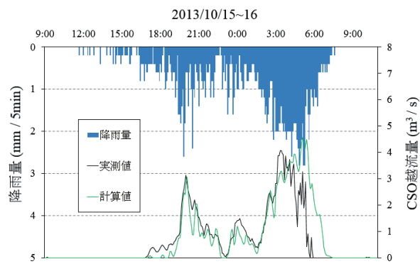
図-9 2013年10月15日～16日の出水を対象としたCSO越流の実測値と計算値の比較グラフ
