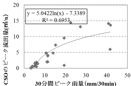
図-7 (c) CSOピーク流出量と30分間ピーク雨量との相関
