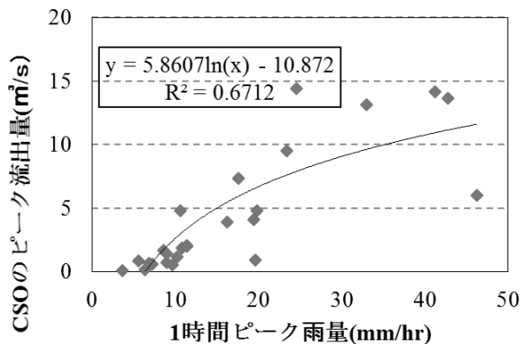
図-7 (d) CSOピーク流出量と1時間ピーク雨量との相関
