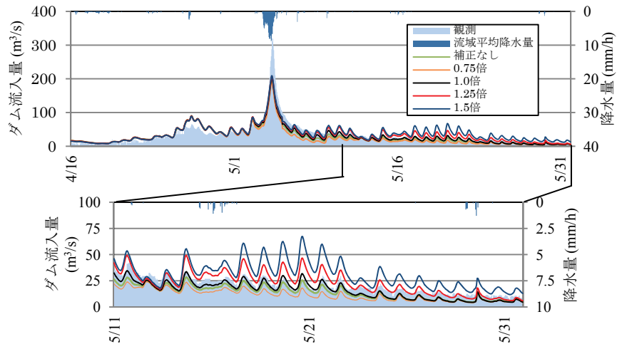
図-7 ダム流入量 (豊平峡ダム・2012年融雪期)
