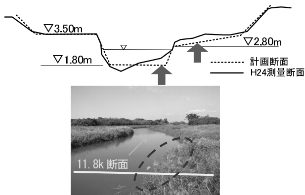
図-5 湿地域C・11.8kの横断図と写真（水路）
