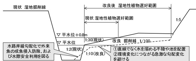
図-13 湿地を維持掘削する場合の留意点
