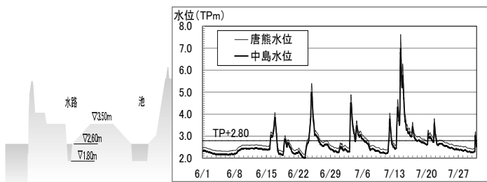
図-3 中島水位と唐熊水位の関係（横断図 12.15km）
