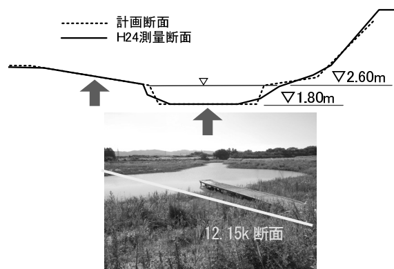
図-6 湿地域B・12.15kの横断図と写真（池）
