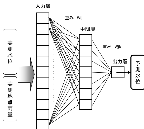
図-2 ニューラルネットワークモデル基本構造
