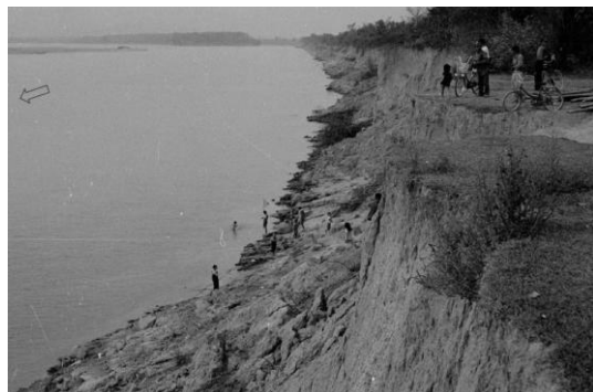
写真-1 河岸侵食の全景 (1998年2月)
