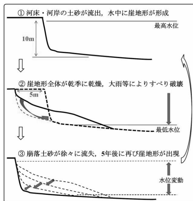
図-3 水位変動に伴う河岸侵食サイクル
