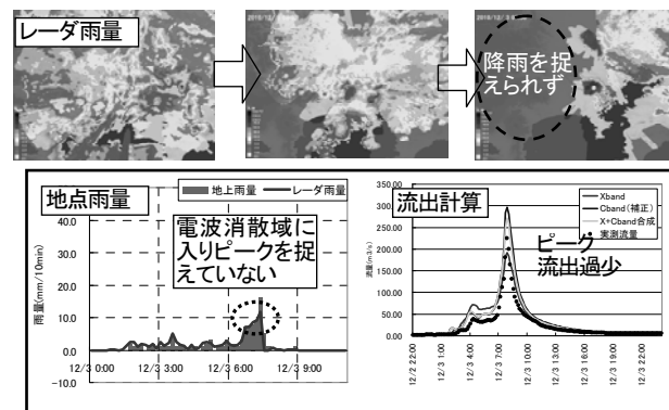
図-6 電波消散による雨量・水位の精度低下(H22. 12降雨事例)
