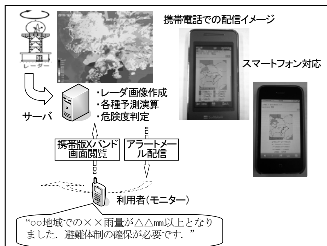
図-2 携帯電話を用いた危険情報配信システム概要
