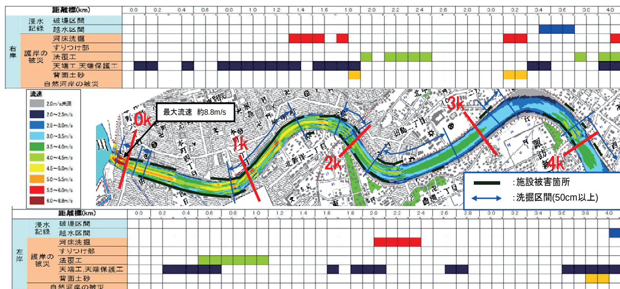
図-7 五十嵐川下流部の流速分布と被災箇所
