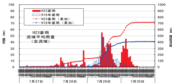
図-2 五十嵐川流域平均雨量 (H. 23, H. 16)
