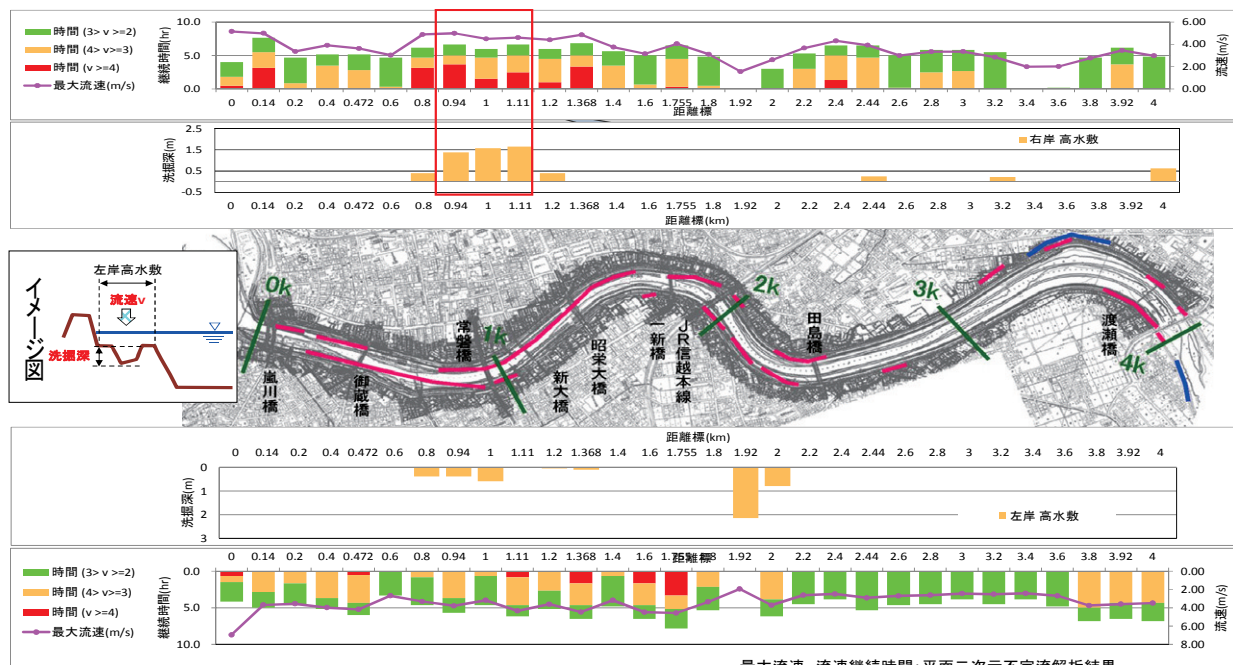
図-8 五十嵐川下流部の流速継続時間と高水敷洗掘深
