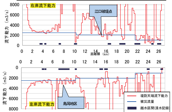
図-6 五十嵐川流下能力と被災流量、越水・破堤箇所
