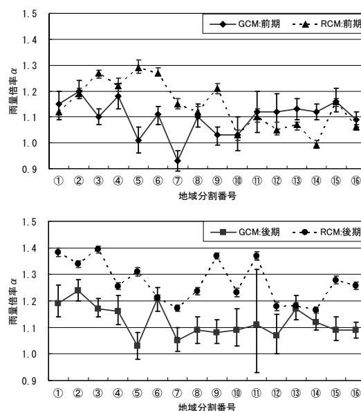
図-5 各気候予測モデルによる雨量倍率(将来)
