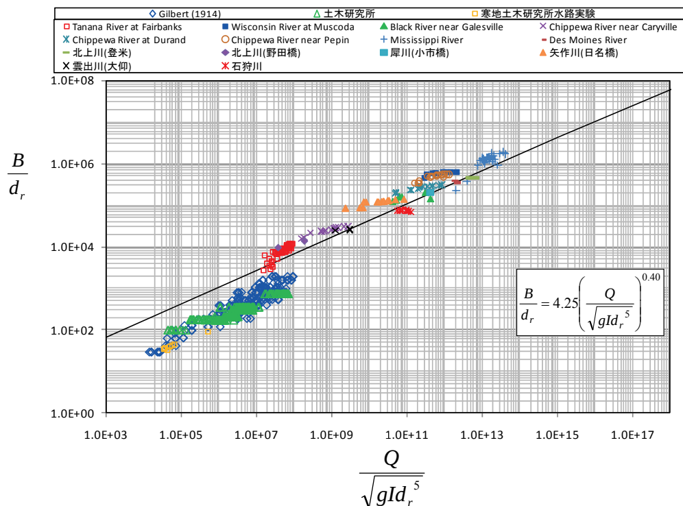
図-3 無次元流量と無次元河幅の関係 8)
