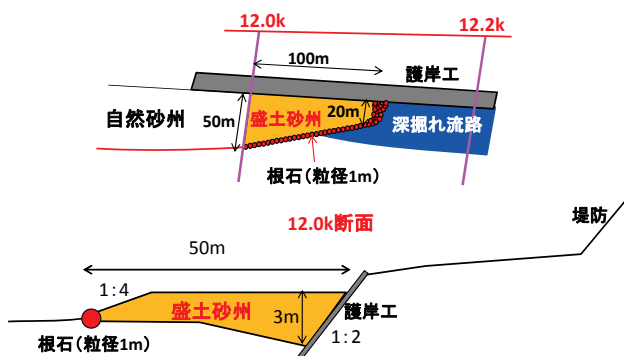
図-11 巨石付き盛土砂州の縦横断面形状 (12.0kの100m案を例に)
