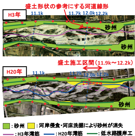
図-9 巨石付き盛土砂州の設置位置・平面形状の決め方
