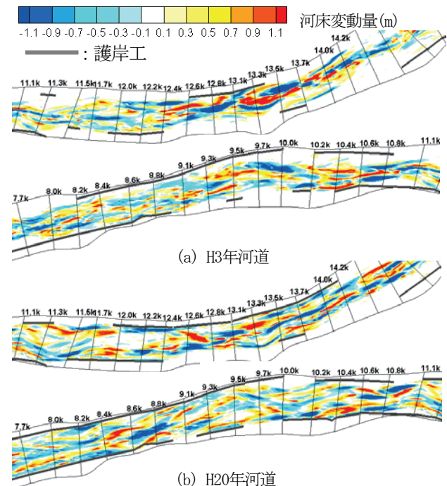
図-7 解析による各断面形の河床変動
