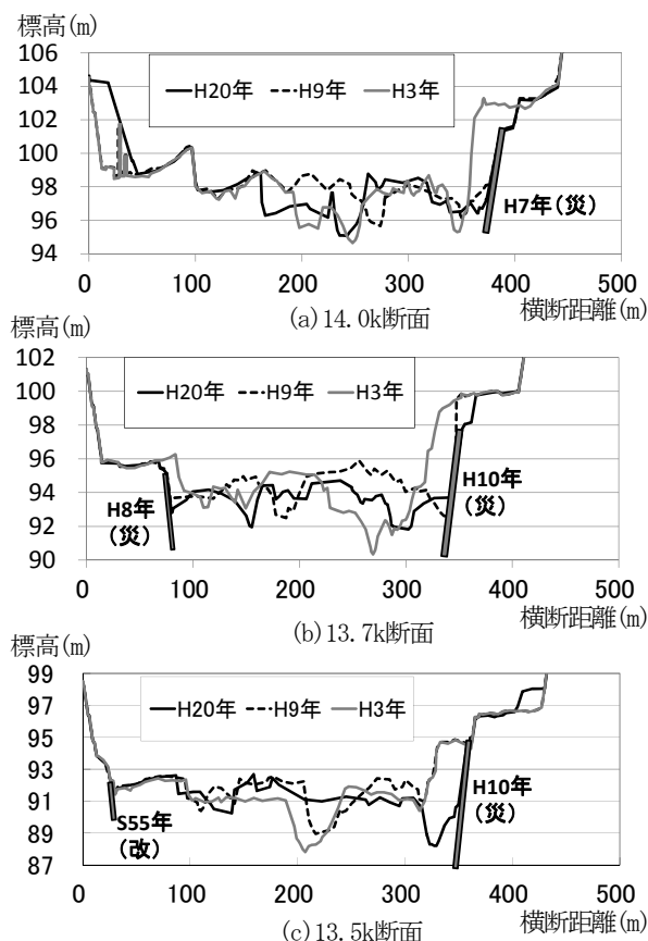
図-8 13.5k～14.0kの横断経年変化
