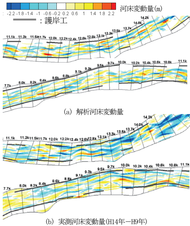
図-5 河床変動量の比較
