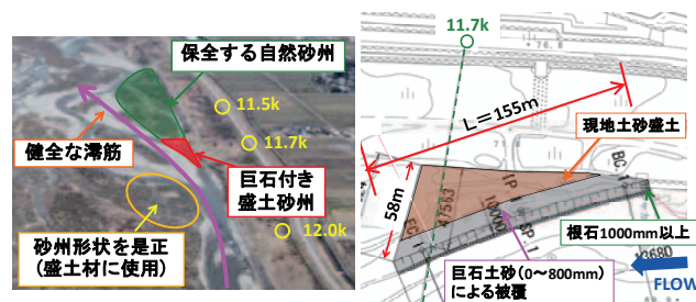
(a) 11.7kの巨石付き盛土砂州の施工計画
