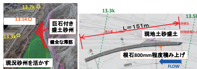
(b) 13.5kの巨石付き盛土砂州の施工計画
