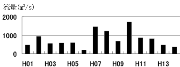
図-1 年最大流量
