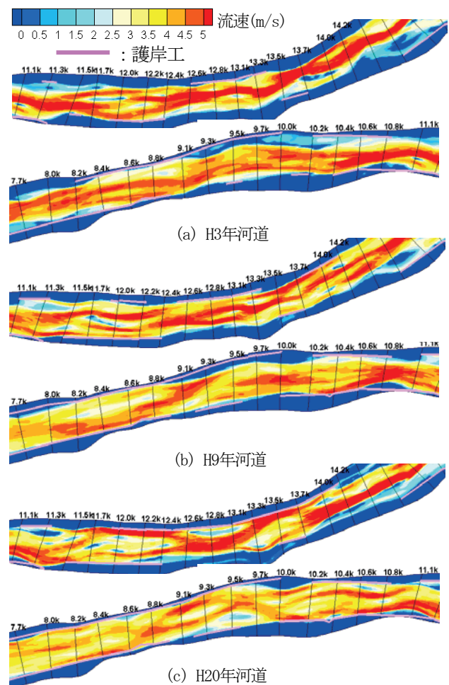
図-6 流速分布の経年変化(洪水流量ピーク時の比較)
