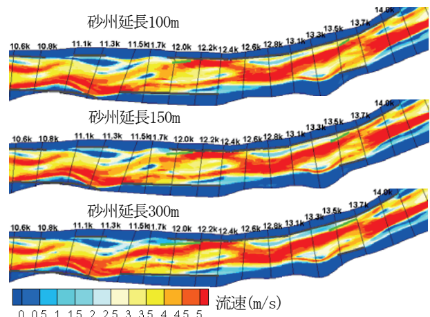
図-12 巨石付き盛土砂州を設置した場合の流速分布
