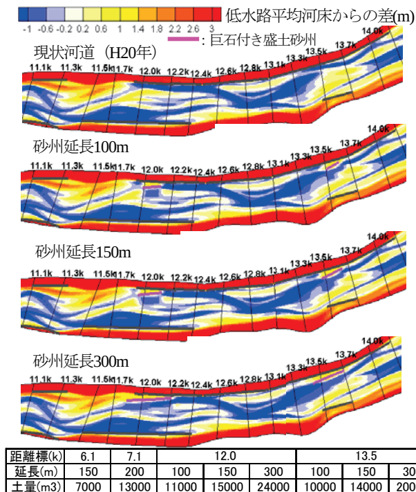
図-10 巨石付き盛土砂州案の河床形状と盛土量
