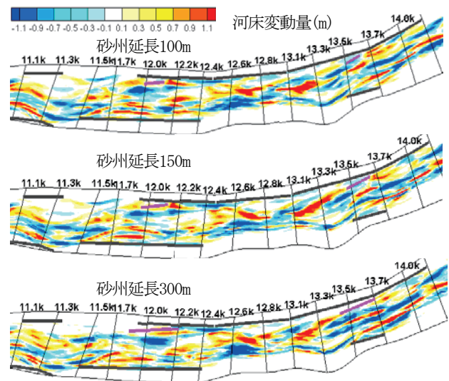
図-13 巨石付き盛土砂州を設置した場合の河床変動
