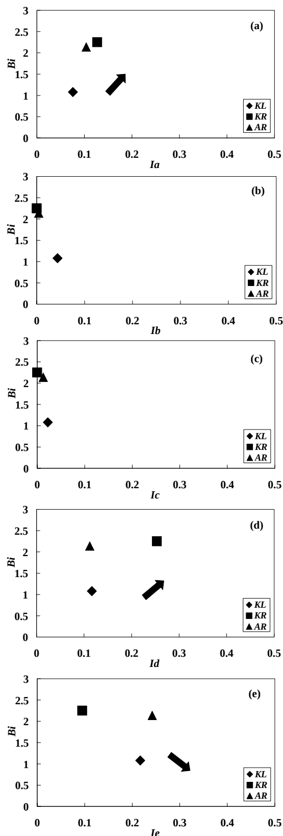
図-6 荒川3砂礫州における各領域の洪水攪乱指標 I_i と生物多様度 BI の関係 (a) Region A, (b) Region B, (c) Region C, (d) Region D, (e) Region E
