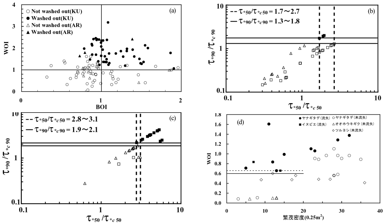
図-4 樹木・草本類の流失限界 WOI の値 \beta , \gamma の検証
