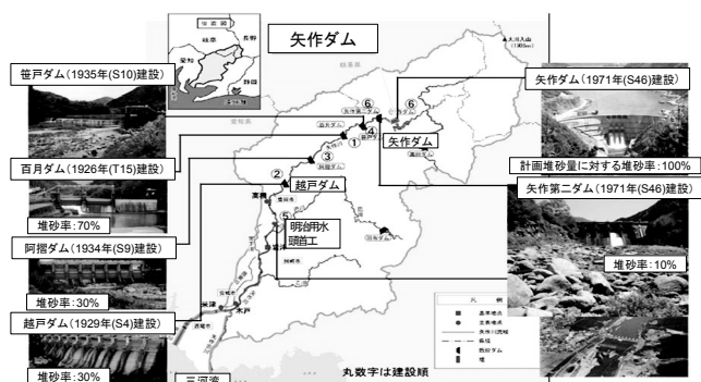
図-2 矢作川流域の土砂還元に関わる主な施設 2)
