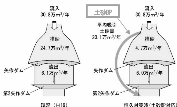
図-3 矢作ダムにおける土砂収支と土砂BPの効果 2)
