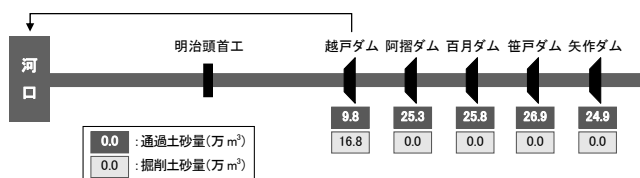
図-8 土砂BP供用後の土砂の通過と堆積状況
