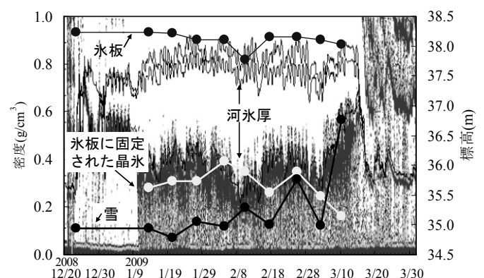
図-7 晶氷厚と密度の変化
