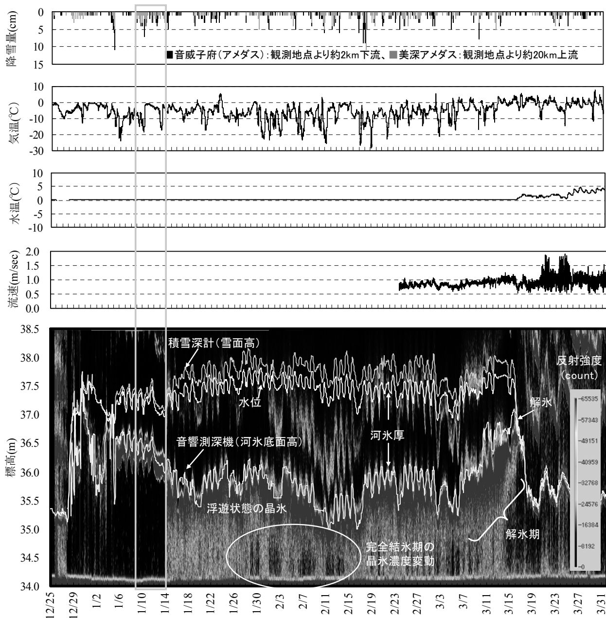
図-5 氷板底面高、晶氷厚、SWIP後方散乱強度コンター
