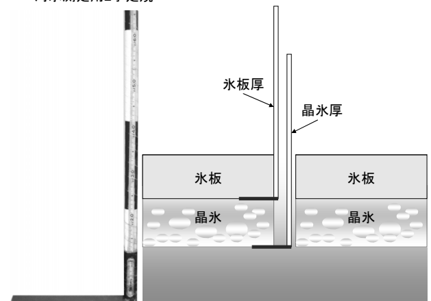
図-4 河氷・晶氷の概要
