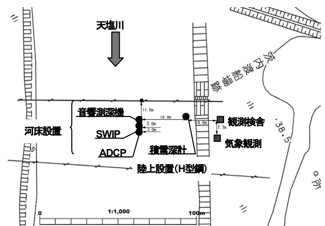
図-2 観測機器の平面配置図
