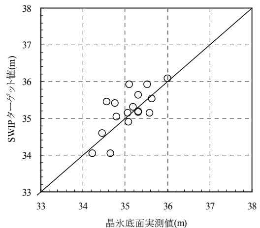
図-6 SWIPの精度検証
