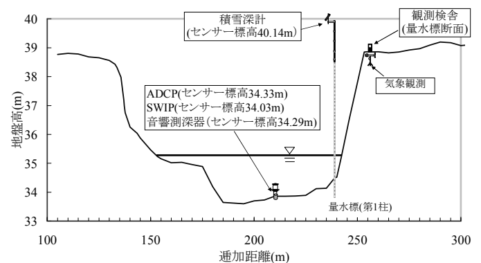
図-3 観測機器の横断配置図
