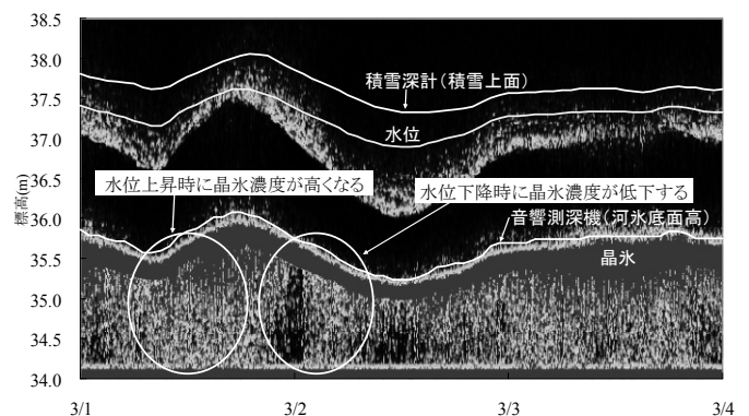
図-8 晶氷厚と水位の変化
