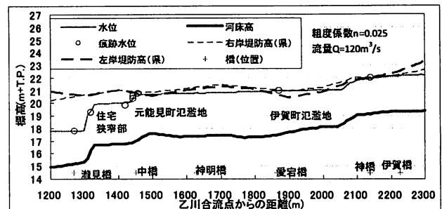
図-10 水位縦断の再現計算と痕跡水位の比較 ( Q=120\text{m}^3/\text{s} 、 n=0.025 を仮定)
