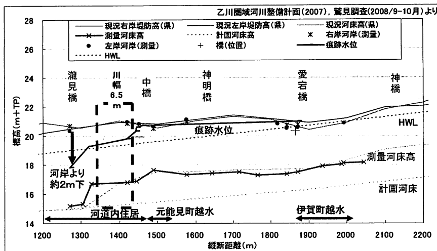
図-3 縦断面図 (痕跡水位, 河床高測量)
