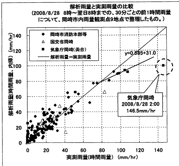
図-8 レーダー・アメダス解析雨量と地点雨量の比較
