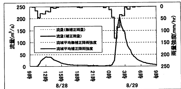
図-9 貯留関数法による計算の例
