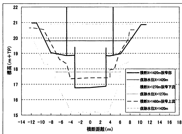
図-4 横断面図 (測量結果, 中橋周辺)
