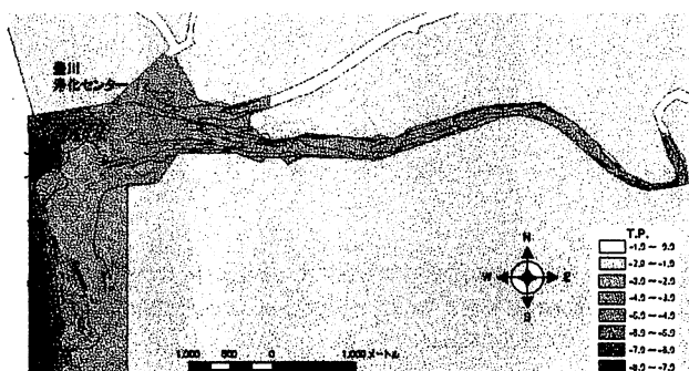
図-3 等深線図
