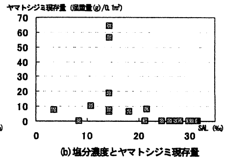
図-10 塩分濃度と現存量
