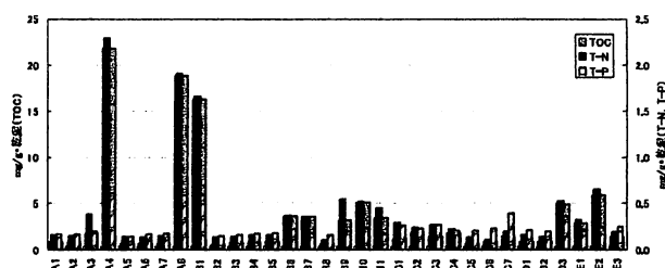
図-5 底質結果
