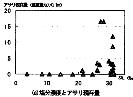
図-10 塩分濃度と現存量
