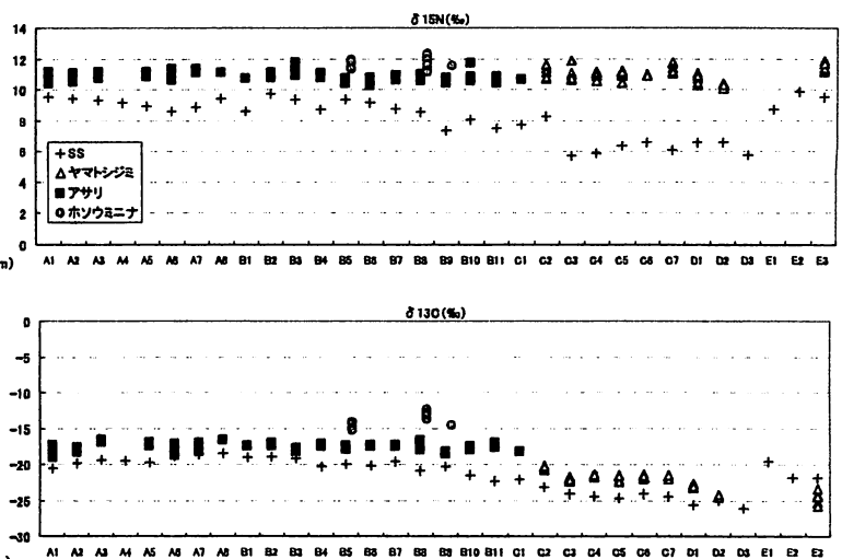
図-8 安定同位体比
