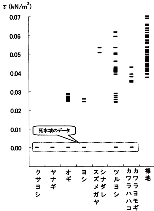
図-8 植物群の立地に働いた推定掃流力 (2000m³/s)
