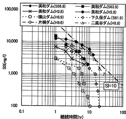
図-8 自然河川におけるSS濃度～継続時間の観測例
