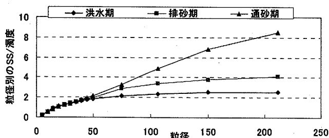
図-13 各粒径階までのSSと濁度の比率 (2005年連携排砂・通砂(宇奈月ダム下流)) 13)
