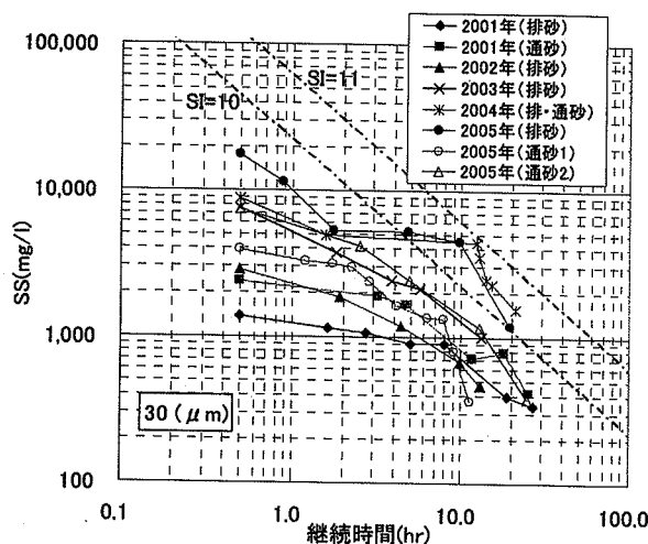
図-11 FSS濃度（ 30\mu\text{m} ）～継続時間の関係
