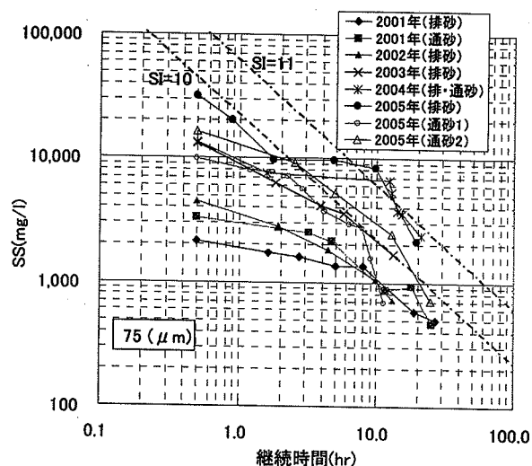
図-10 FSS濃度（ 75\mu\text{m} ）～継続時間の関係
