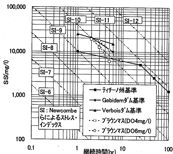
図-7 既往のダム排砂時のSS濃度基準
