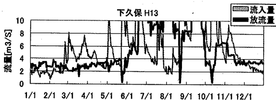
図-9 富郷、新宮、下久保ダムの流入量と放流量
