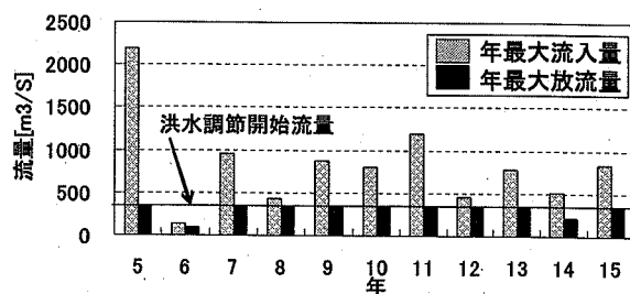
図-5 下笠ダムにおける年最大流入量と放流量
