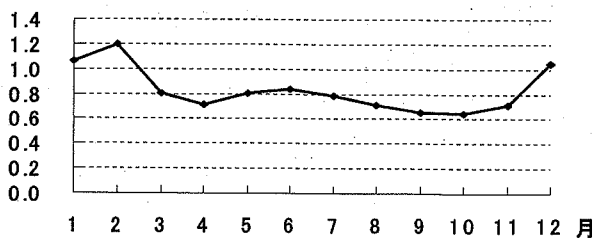
図-15 月別最大放流量の総和／月別最大流入量の総和の平均値
