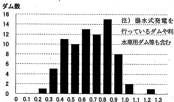
図-1 年最大放流量/年最大流入量のヒストグラム
