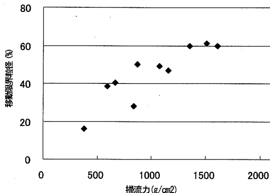
図-16 掃流量と限界粒径の関係
