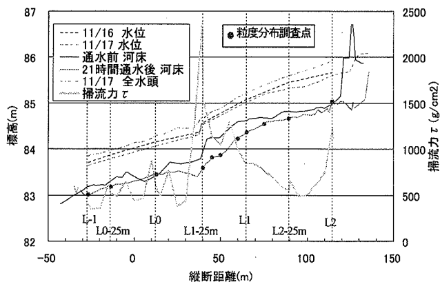
図-14 開削水路の河床高、水位、掃流力縦断分布
