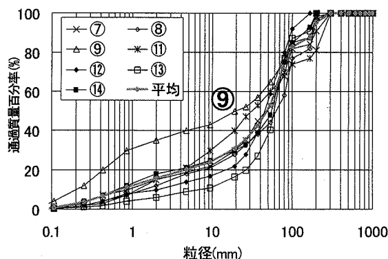
図-12 滞筋部表層下粒度分布(7.1km)
