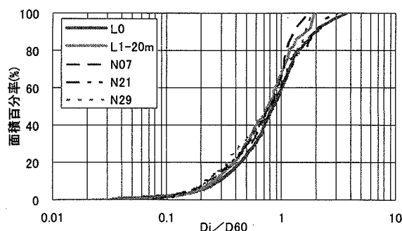
図-17 粒度分布形状の比較
