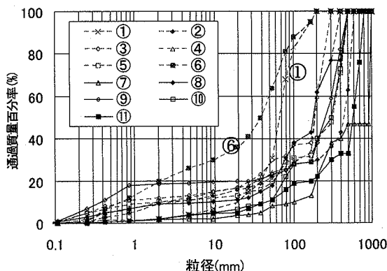
図-10 表層粒度分布(13.1km)
