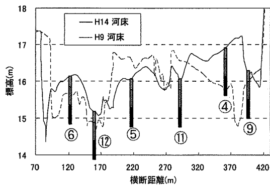
図-11 鉛直・横断採取位置(7.1km)
