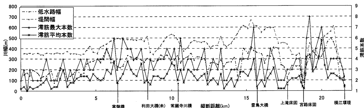
図-5 滞筋本数の縦断分布 (平成3年～平成14年)
