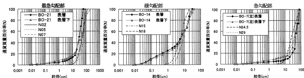
図-18 ふるい分析と画像分析の比較
