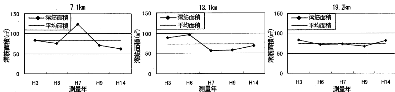
図-6 滞筋面積の変動
