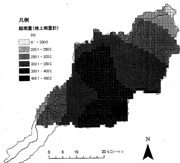
図-5 総雨量（地上雨量計）の分布．八田 4) により作成された総雨量分布図をメッシュ単位に再加工．
