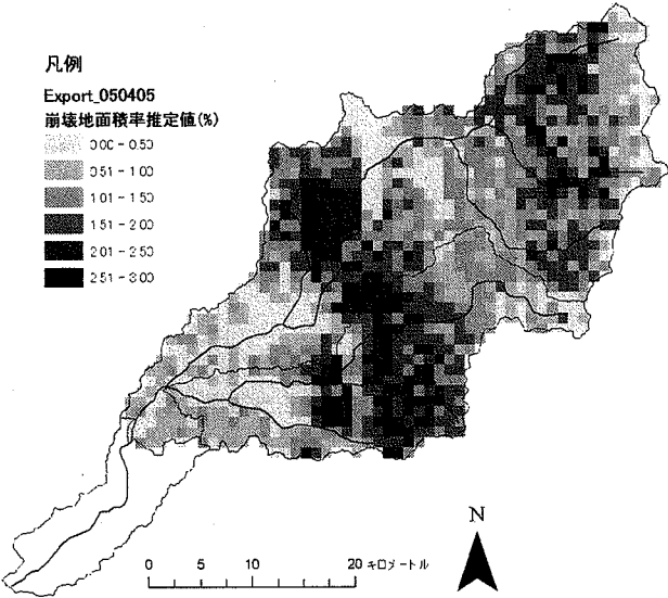
図-8 崩壊地面積率の推定結果(二風谷ダム上流域)
