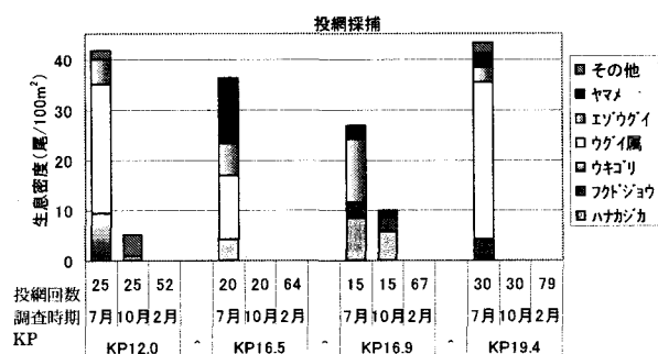
図-9 調査地点別の生息密度(投網)
