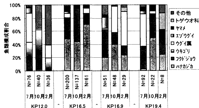
図-8 調査地点別魚類構成割合
