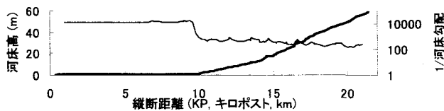
図-1 豊平川の河床縦断面図
