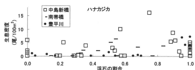
図-20 浮石とハナカジカの分布(2002.2)
