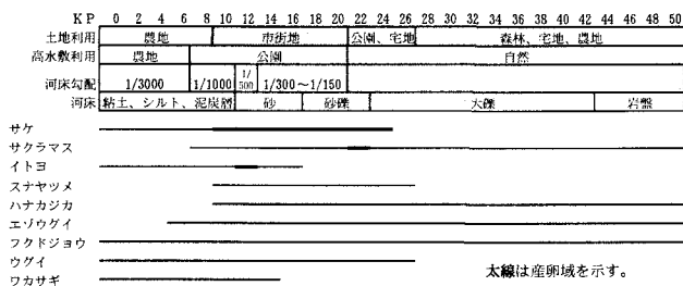
図-7 豊平川における魚類の縦断分布
