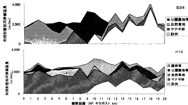
図-4 豊平川河岸線の利用形態別延長の変遷
