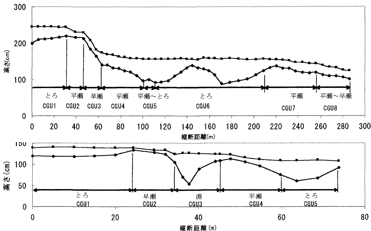
図—2 河床及び水位の縦断面図 上：川浦川 下：北川
