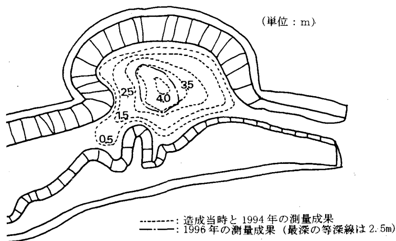
図－３．人工わんど広拡部の水深の変遷
