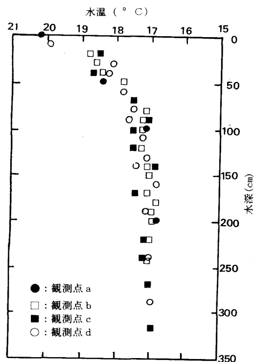
図－４．水温の水深方向の分布
