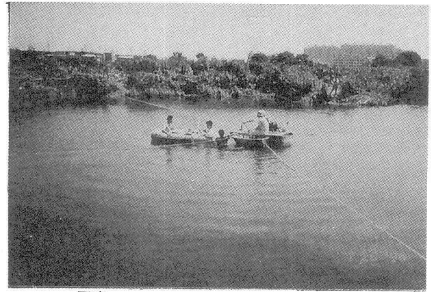
写真－２．ADCP による流速分布測定
