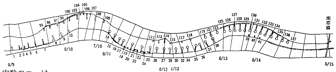
図 - 1 長期 20 ヶ年河道改修計画案
