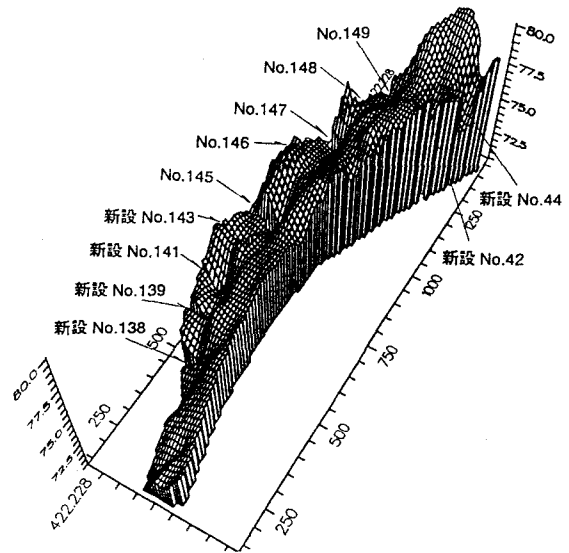
図 - 12 新設水制設置後（計画）河床鳥瞰図
