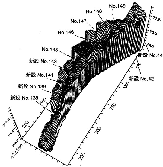
図-11 新設水制設置後 (融雪後) 河床鳥瞰図
