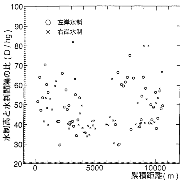
図-4 水制高と水制間隔との関係
