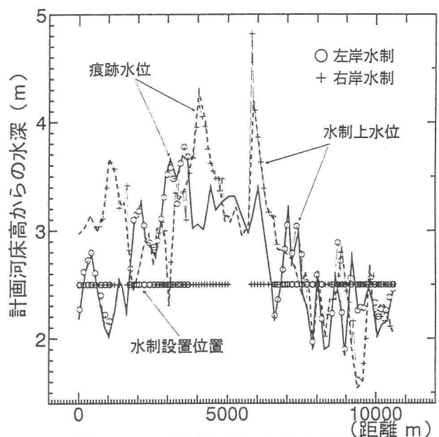
図-3 水制設置による水位変化
