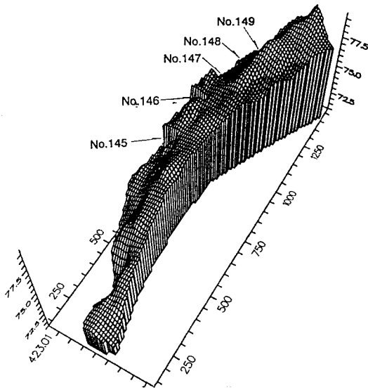
図-10 既設水制融雪後河床鳥瞰図
