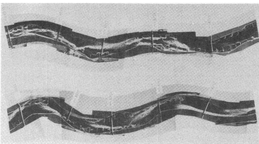
写真-3 計画高水流量流下後の河床状態
