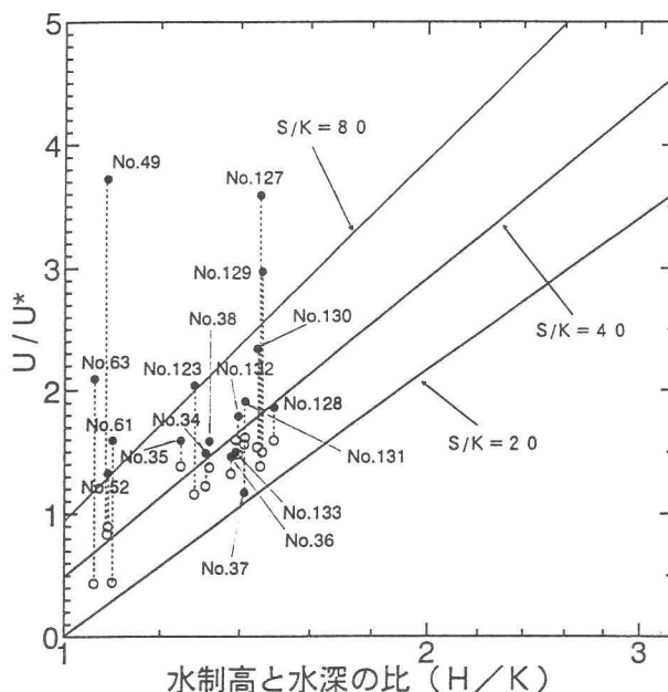
図 -7 水制の抵抗 ( u/u^*H )
