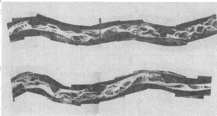
写真-2 初期河床状態（融雪流量流下後）
