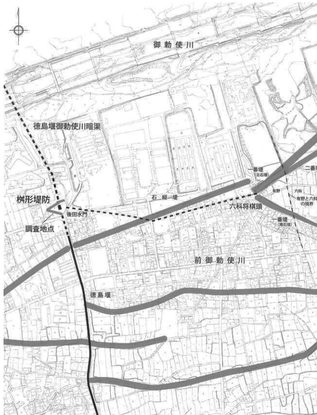
図 11・後田櫛形堤防周辺地形図
