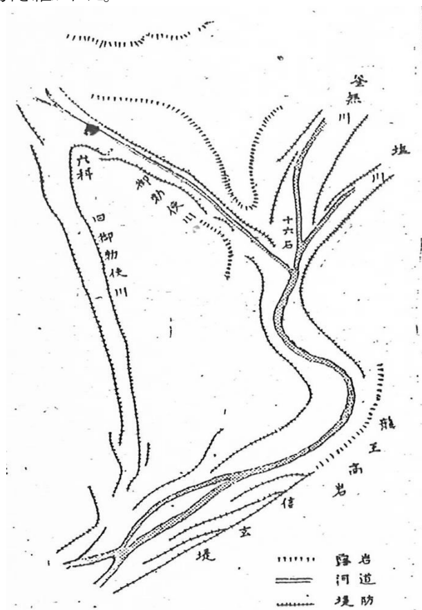
図 13・釜無川と御勅使川の洪水制御のシステム
