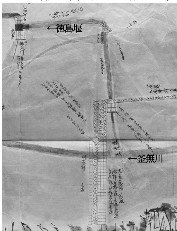
図 2・徳島堰頭首工絵図
