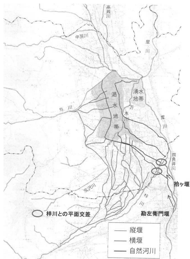
図7・勘左衛門堰と拾ヶ堰
