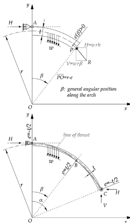
図-11 CCR の解析の概念図 (CCR の論文の Fig.9, 10)
