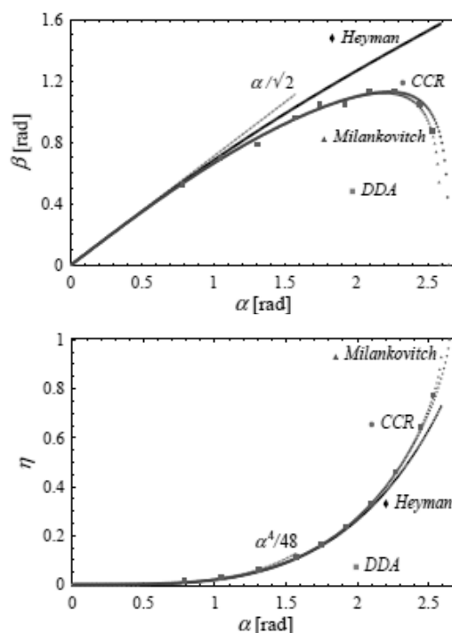
図-12 Heyman, CCR, ミランコビッチ理論及び DDA 解析結果の比較 9) (上:破壊角,下:無次元厚さ)
